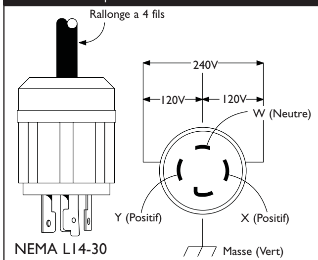
Figure 26 – Prise à Verrouillage de 120/240 Volts c.a., 30 Ampères
