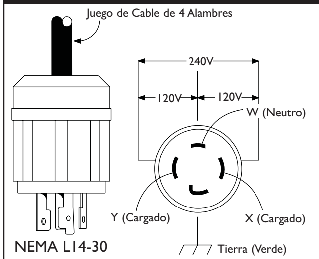
Figura 42 — 120/240 Volt AC, 30 Amp, Receptáculo de Seguridad
