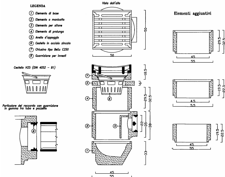
Figura 40.2. – Esempio di caditoia stradale in cls vibrato con chiusino Be Gu (con accumulo di fanghi e sifone)
