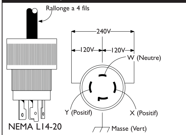
Figure 22 – Prise à Verrouillage de 120/240 Volts c.a., 20 Ampères
