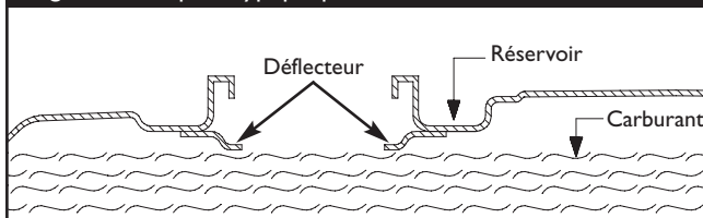
Figure 16 - Espace Typique pour la Dilatation du Carburant
