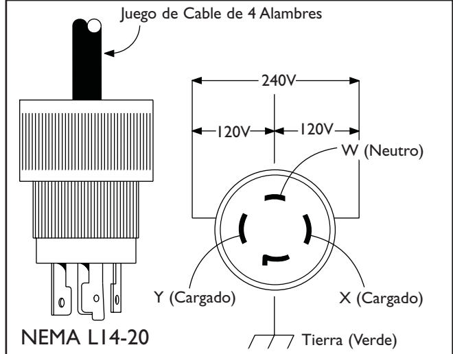
Figura 36 — 120/240 Volt AC, 20 Amperios, Receptáculo de Seguridad
