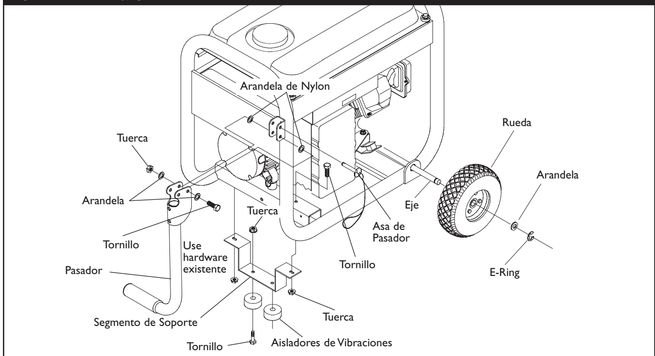
Figura 29 — Instale el Juego de Ruedas
