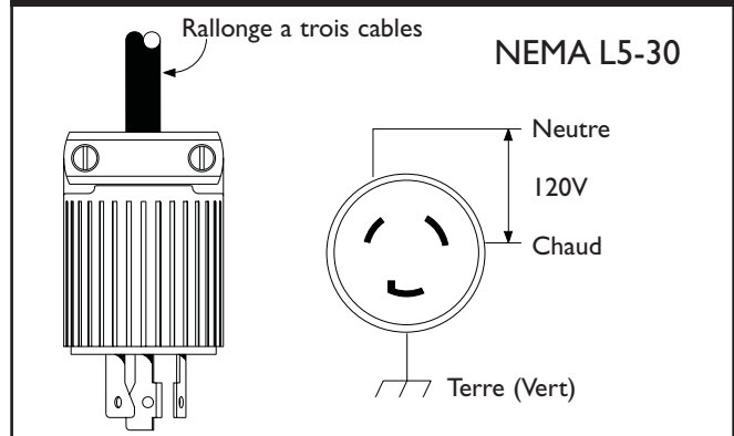
Figure 23 - Prise à Verrouillage de 120 Volts c.a., 30 Ampères
