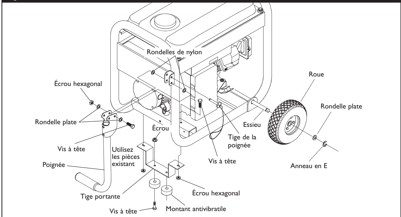
Figure 15 — Installe la roue la trousse
