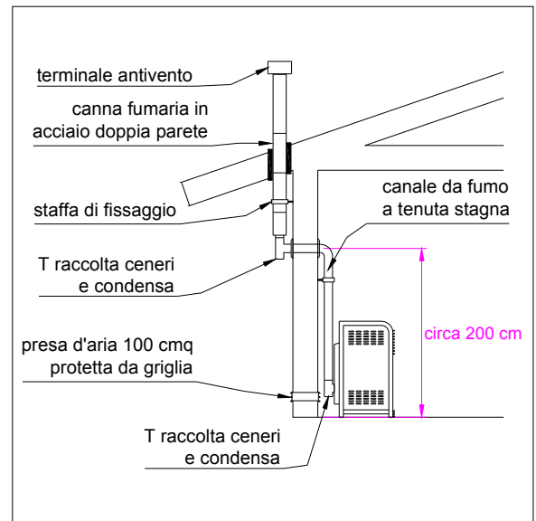
b2) canna fumaria a doppia parete esterna con canale da fumo interno (a tenuta stagna)
