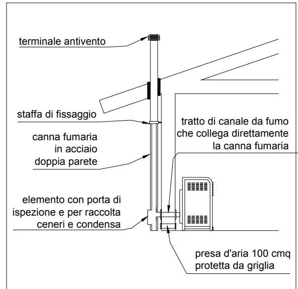
b1) canna fumaria a doppia parete esterna
