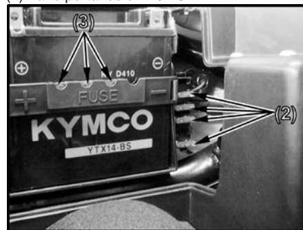
(2) Fusibili 10-15 A
