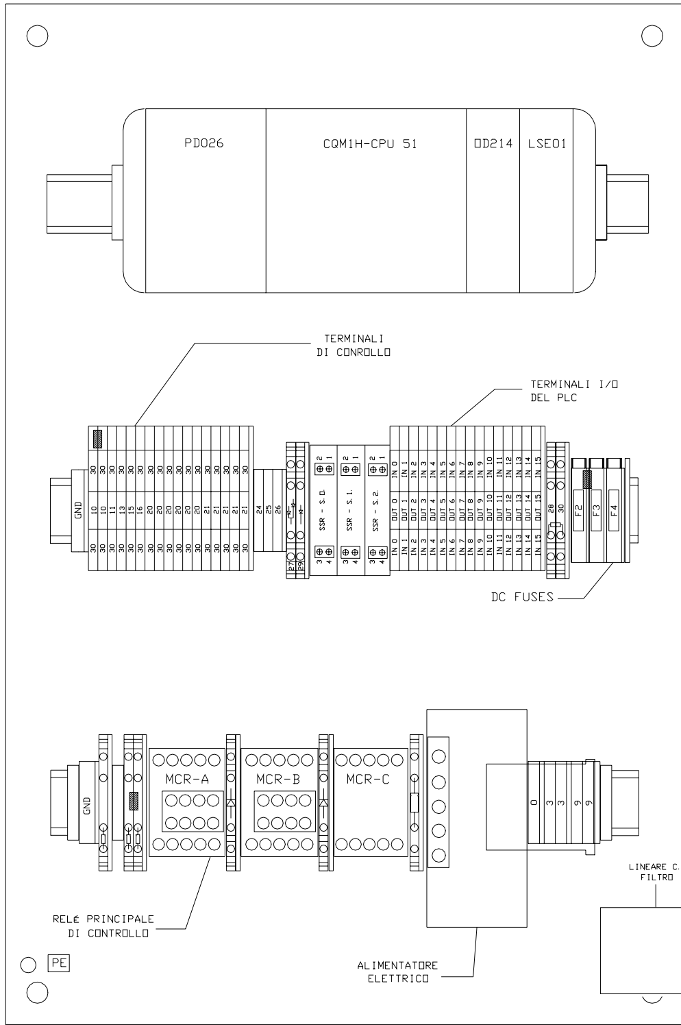
FIGURA 8-1 DISPOSIZIONE DELL' ARMADIO ELETTRICO
