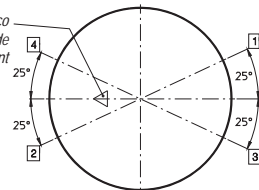
Posizione chiusura segmenti Position of piston ring closing / Position fermeture segments
