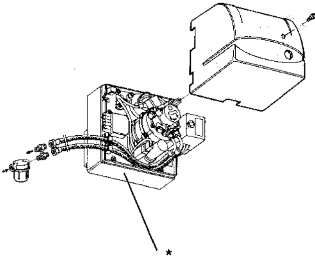
MOTORE AACO
