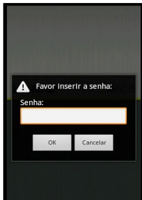
Login
