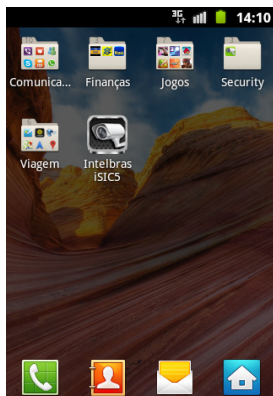
Aplicativo iSIC 5
