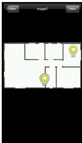
Mapa configurado
