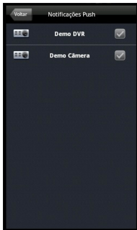
Notificações Push
