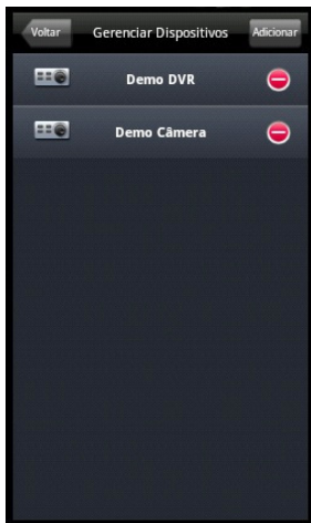
Gerenciar dispositivos
