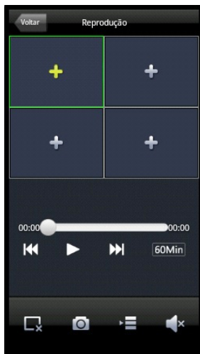
Reprodução
