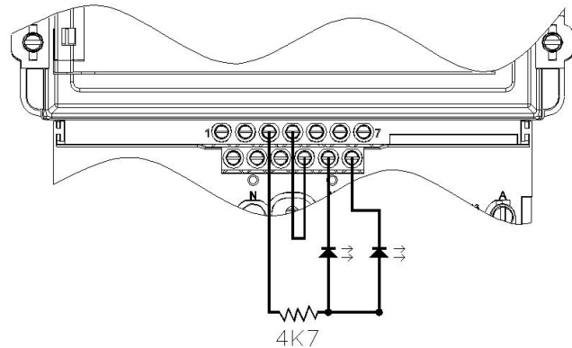
Figura 3.11 – Sugestão para avaliação das saídas de pulsos KYZ do ELO2173.
