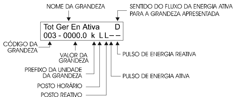
Figura 5.1 – Mostrador no modo Normal do ELO2173.
