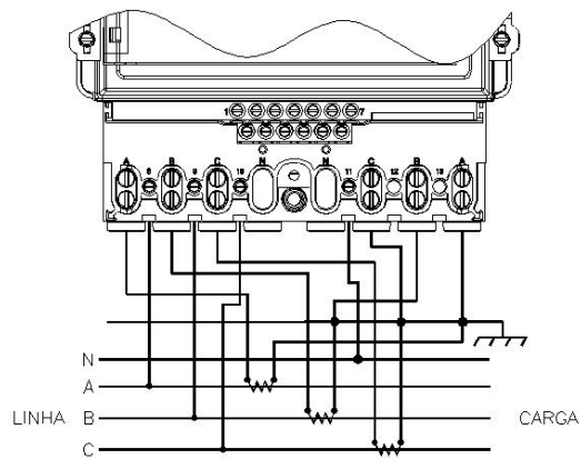
Figura 3.9 - Medição a 3 elementos estrela direta em tensão (sem TPs) e indireta em corrente (3 TCs) do ELO2173.
