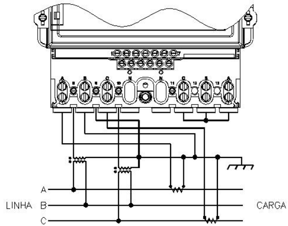
Figura 3.8 - Medição a 3 elementos com 2 TPs e 2 TCs do ELO2173.
