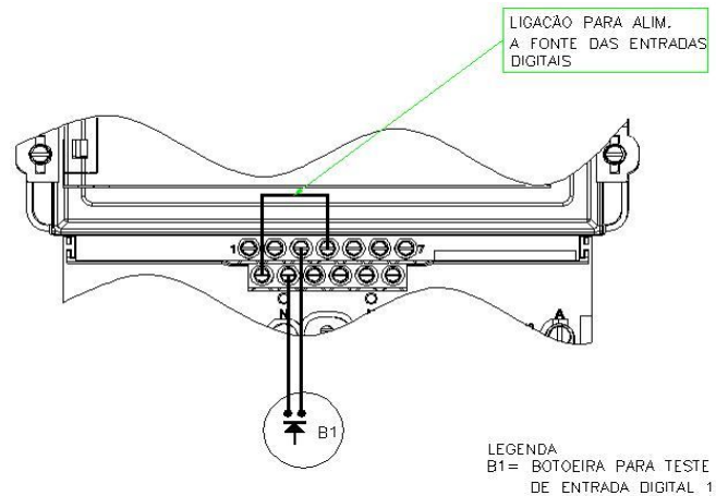
Figura 3.13 – Sugestão para avaliação das Entradas Digitais do ELO2173.
