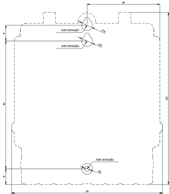
Figura 3.2 – Medidas para instalação do ELO2173.
