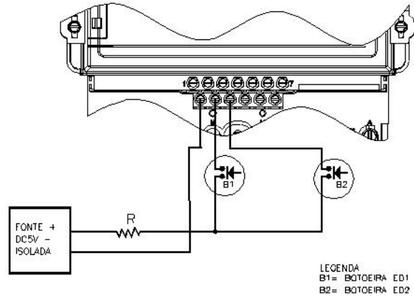
Figura 3.12 – Ligação para aplicação das Entradas Digitais do ELO2173.
