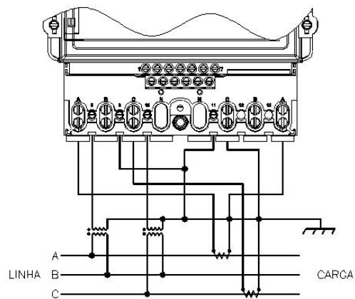
Figura 3.5 - Medição a 2 elementos com 2 TP e 2 TC (Ligação Delta Aberto) do ELO2173.
