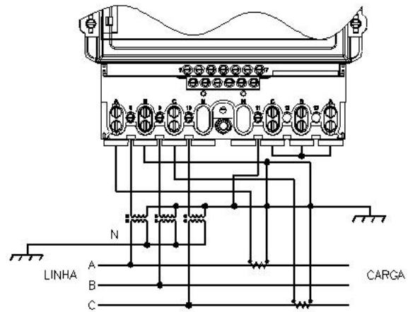
Figura 3.7 - Medição a 3 elementos com 3 TPs e 2 TCs do ELO2173.
