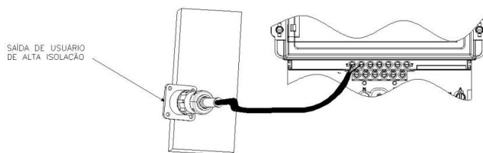
Figura 3.10 – Conexão da saída de usuário do ELO2173 através de um cabo de alta isolamento (óptico).
