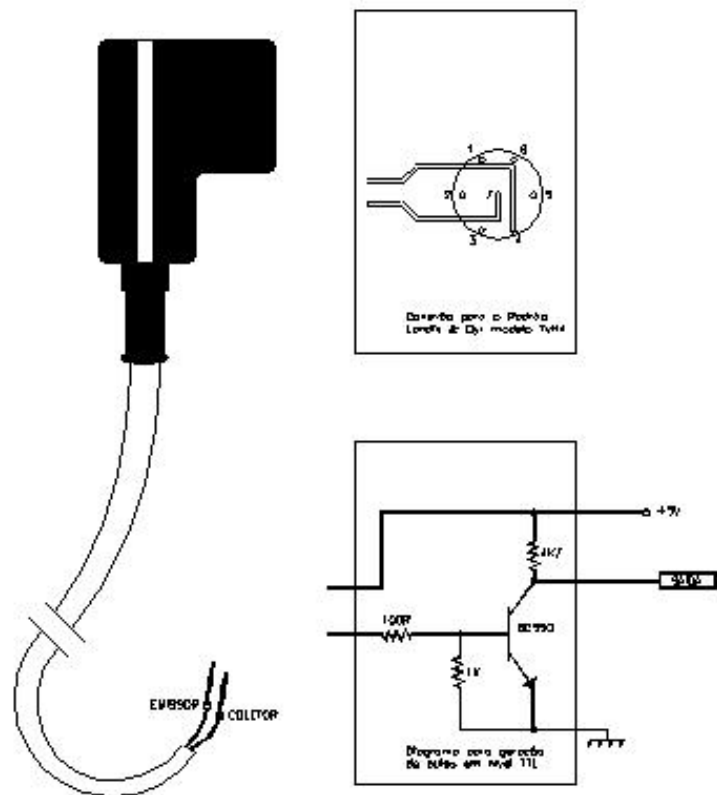
Figura 7.1 - Conexão do cabo de captura de pulsos.
