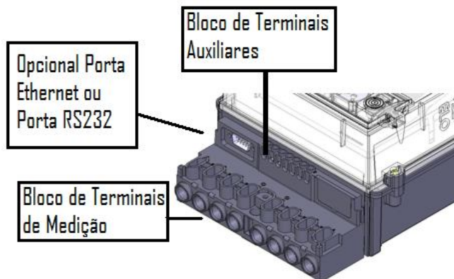
Figura 2.3 – Conectores e Blocos de terminais do ELO2173.
