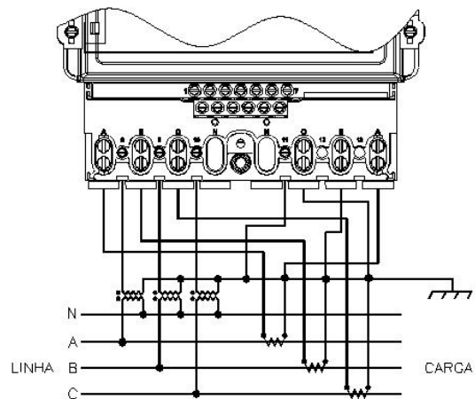
Figura 3.4 - Medição a 3 elementos com 3 TP e 3 TC (Ligação Estrela) do ELO2173.
