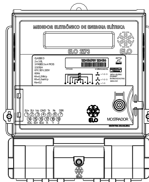
Figura 2.4 – O painel frontal e informações do medidor ELO2173
