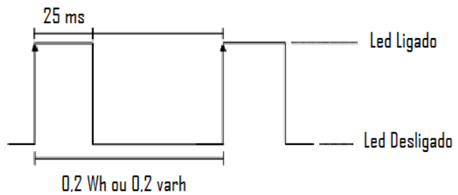
Figura 7.2 - Forma de onda dos pulsos de calibração.
