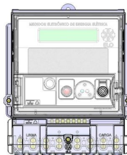
Figura 2.1 - Vista frontal do modelo ELO2173.
