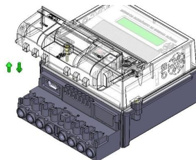
Figura 3.1 – Detalhe da tampa do bloco de terminais do ELO2173.
