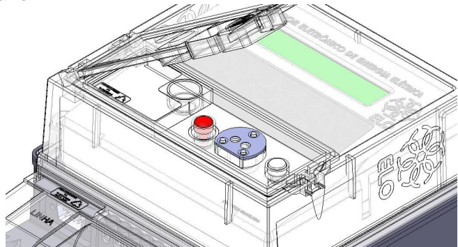
Figura 2.2- Conector magnético para comunicação e botões do ELO2173.
