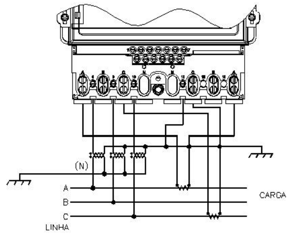
Figura 3.6- Medição a 2 elementos com 3 TPs e 2 TCs do ELO2173.
