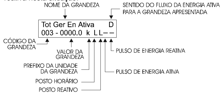
Figura 7.3 – Disposição de informações no mostrador
