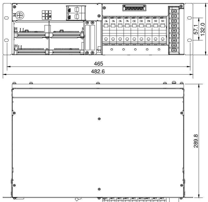
Figura 2-2 Dimensões da Instalação (unidade: mm)
