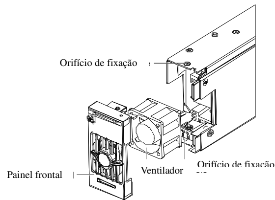
Figura 4-2 Desmontagem do painel frontal
