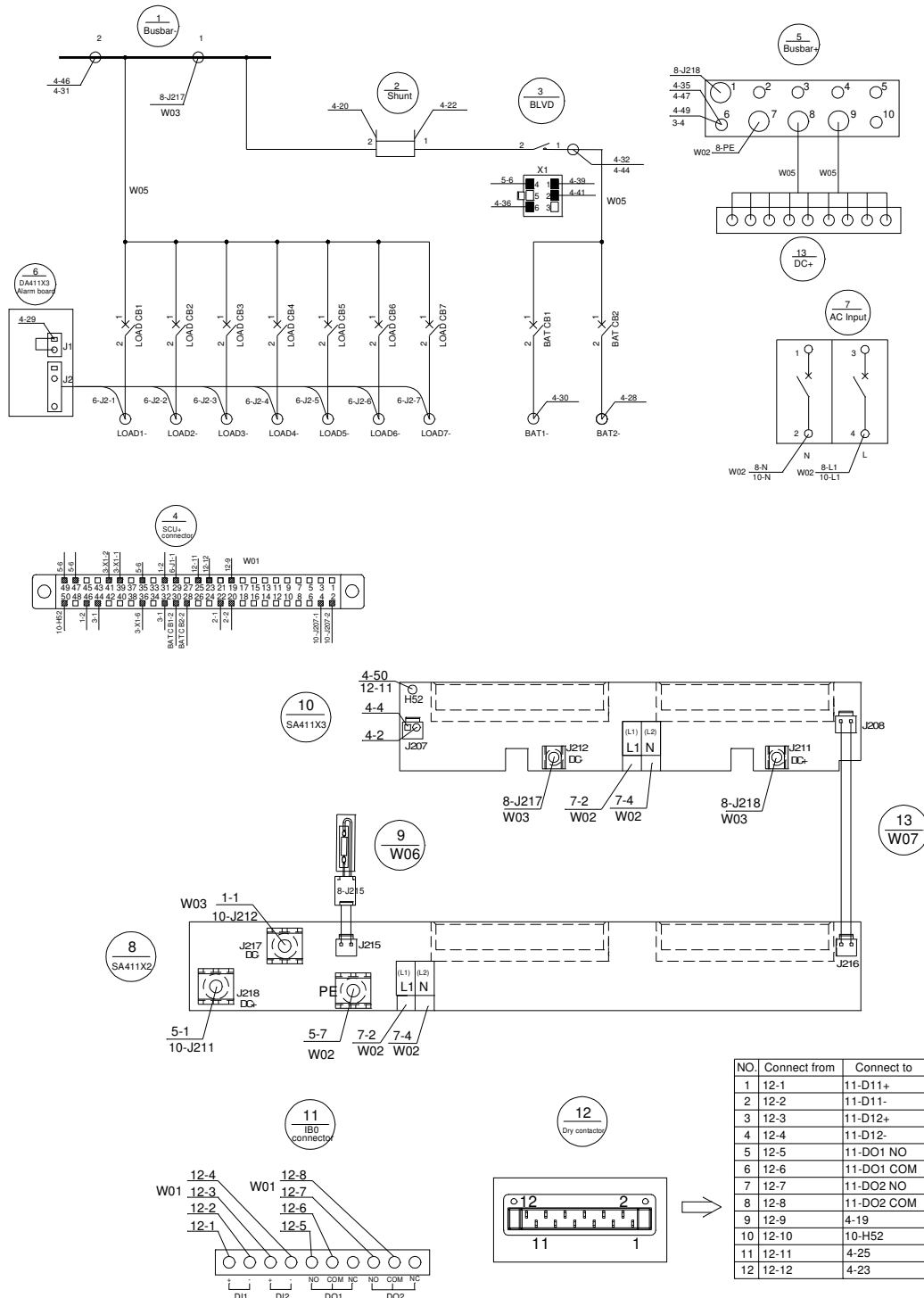
Figura 1 – Diagrama de fiação do sistema
