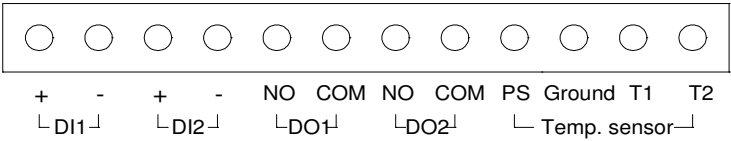
Figura 2-4 Terminal de conexão da sonda DI/DO/temperatura
