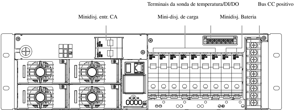
Figura 2-3 Terminais de conexão
