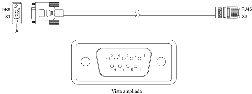
Figura 2-1 Cabo RS232
