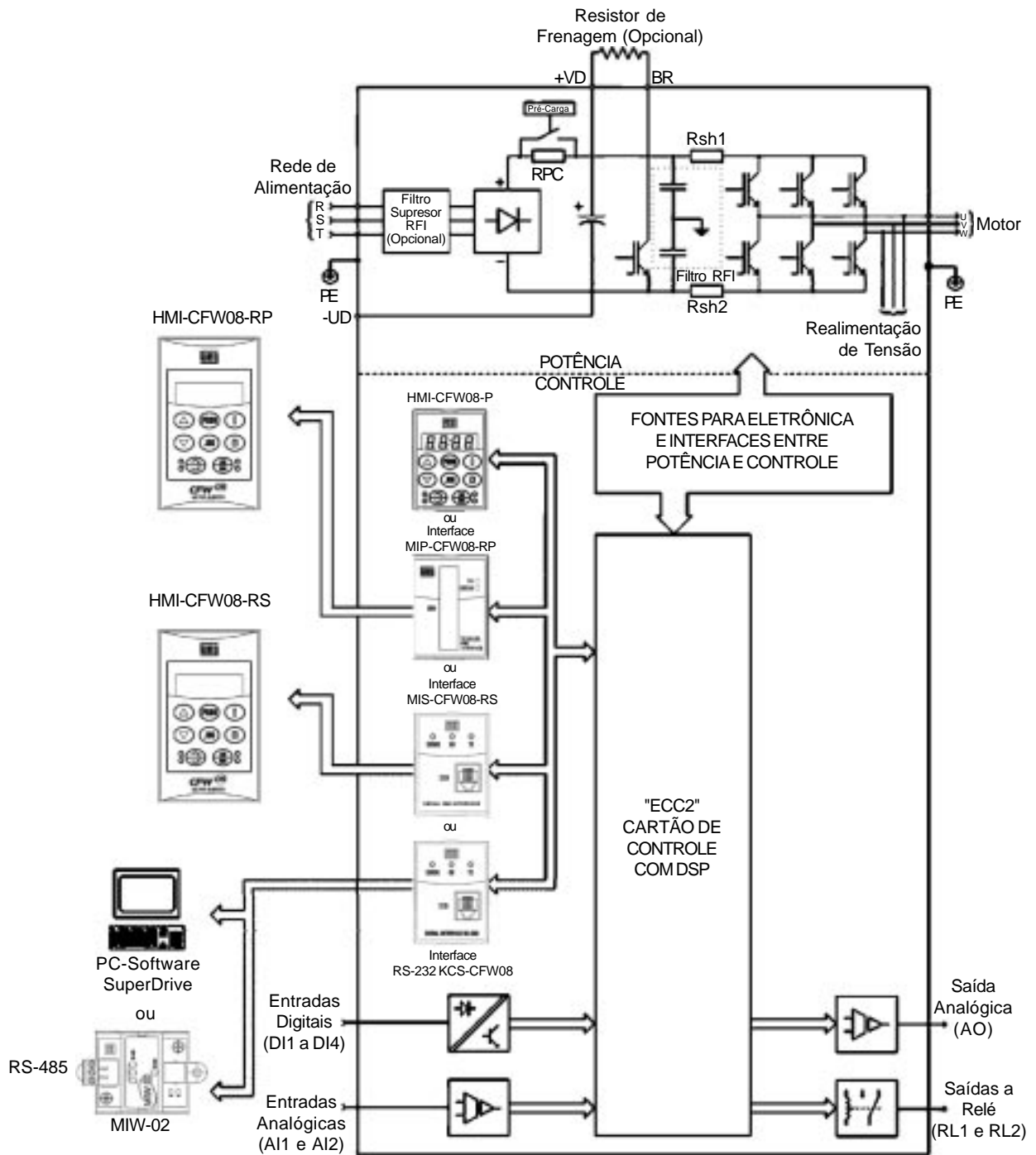
Figura 2.2 – Diagrama de Blocos para os modelos: 7.3-10-16A/200-240V e 2.7-4.3-6.5-10-13-16A/380-480V Obs.: O modelo 16A/200-240V não possui Filtro Supresor de RFI opcional.
