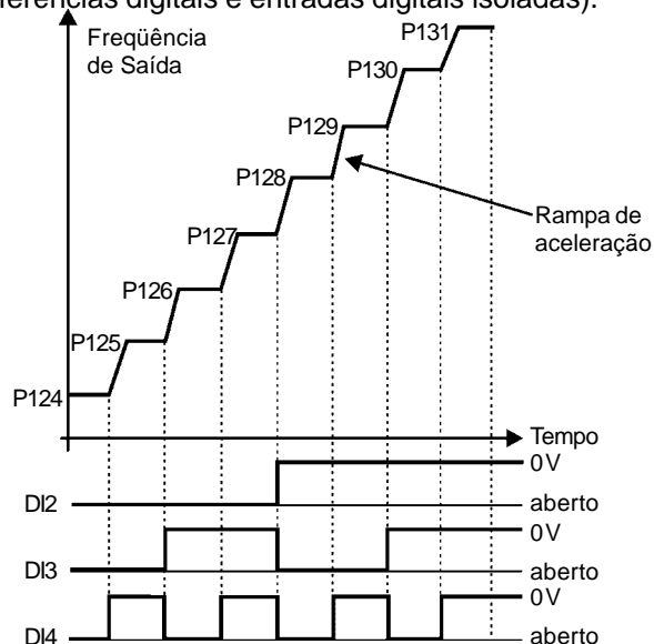
Figura 6.5 - Diagrama de tempo da função multispeed
