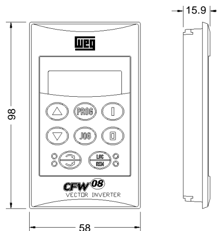
Figura 8.8 - Dimensões da HMI-CFW08-RS
