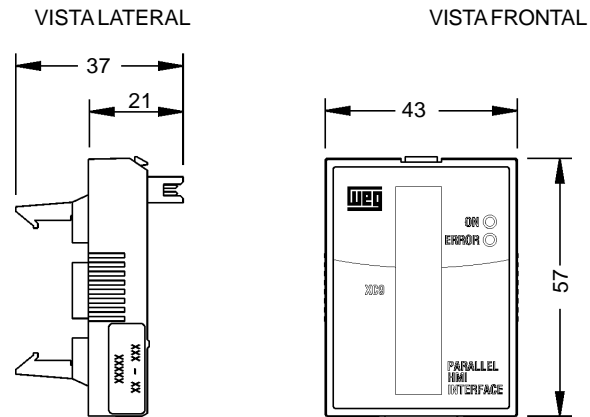
Figura 8.6 - Dimensões da MIP-CFW08-RP
