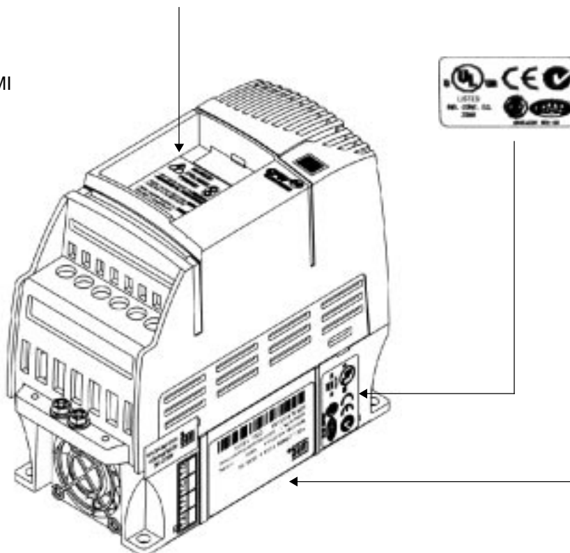
Figura 2.4 - Descrição e localização das etiquetas de Identificação
