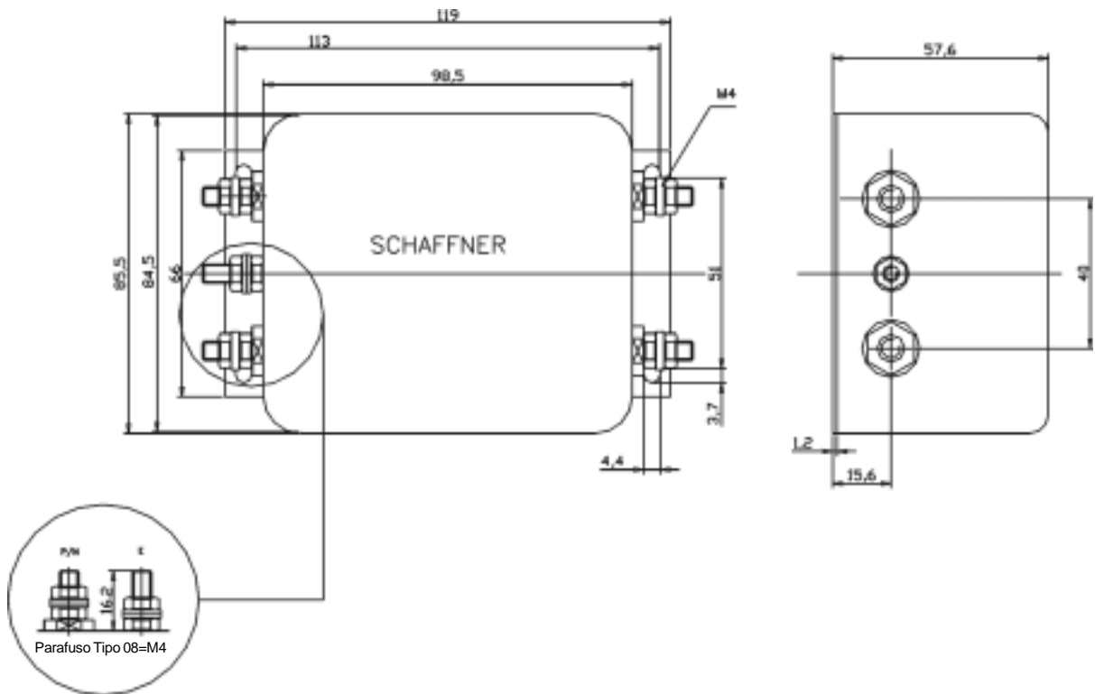
Figura 3.18 - Desenho dos filtros externos FS6007-25-08 e FS6007-36-08
