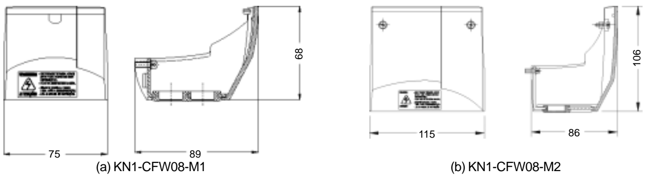
Figura 8.17 - dimensões dos kits NEMA1/IP20
