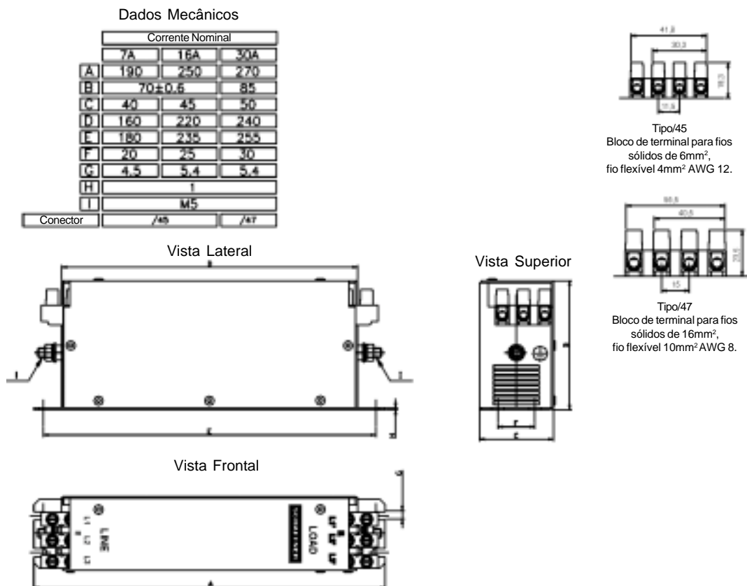
Figura 3.19 - Desenho do filtro externo FS3258-xx-xx
