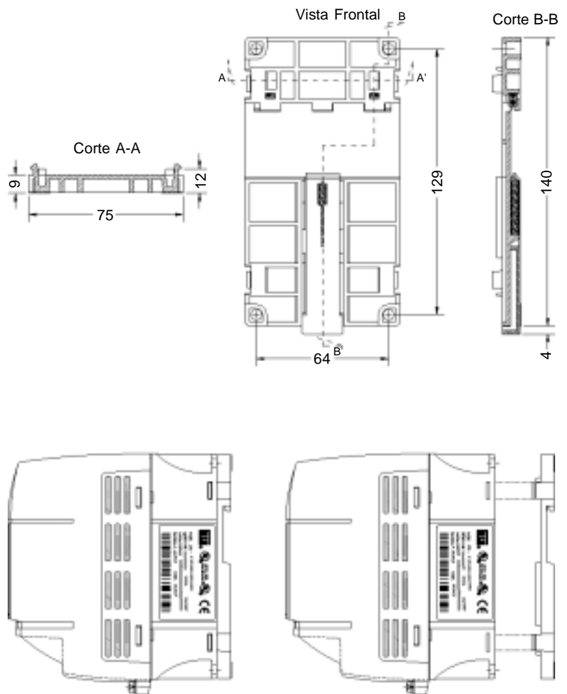
Figura 8.15 - Inversor com kit trilho DIN (KMD-CFW-08-M1)
