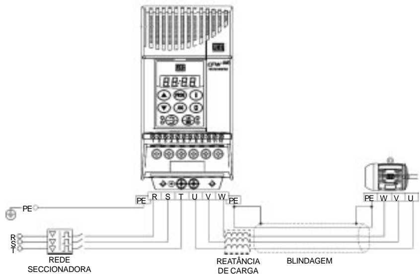
Figura 8.22 - Conexão da reatância de carga
