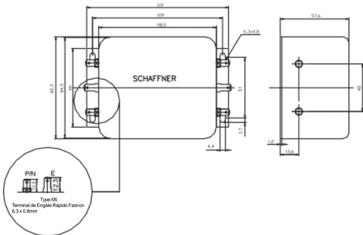
Figura 3.17 - Desenho do filtro externo FS6007-16-06
