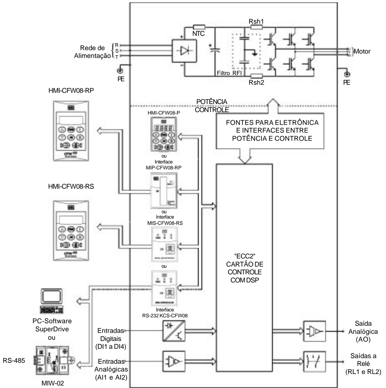
Figura 2.1 - Diagrama de Blocos para os modelos: 1.6-2.6-4.0-7.0A/200-240V e 1.0-1.6-2.6-4.0A/380-480V
