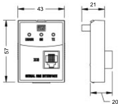
Figura 8.11 - Dimensões do módulo de comunicação serial MIS-CFW08-RS para HMI remota serial
