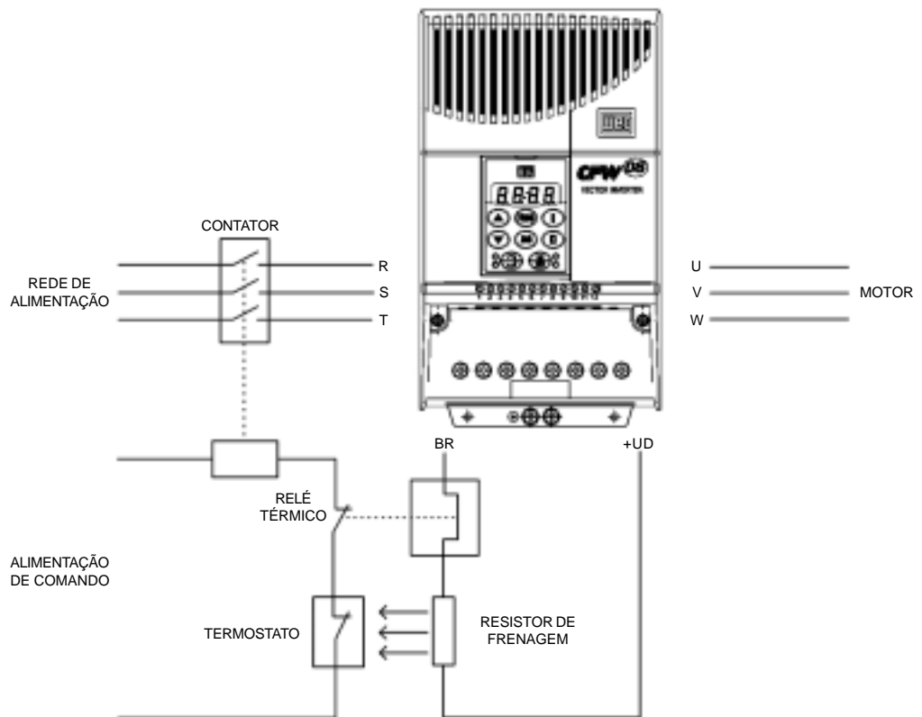
Figura 8.23 - Conexão do resistor de frenagem (só para os modelos 7.3-10-16A/200-240V e 2.7-4.3-6.5-10-13-16/380-480V)
