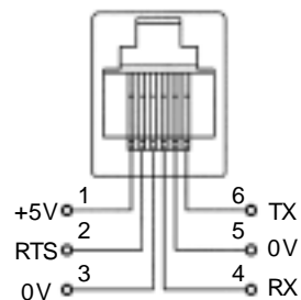
Figura 8.25 - Descrição sinais do conector XC8 (RJ-6)
