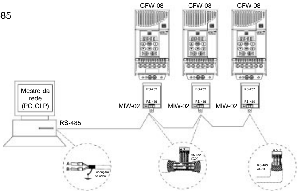
Figura 8.24 - Conexão do CFW-08 em rede RS-485
