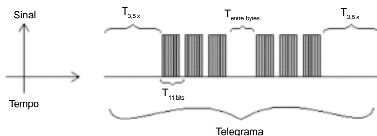
Figura 8.27 - Tempos envolvidos durante a comunicação de um telegrama
