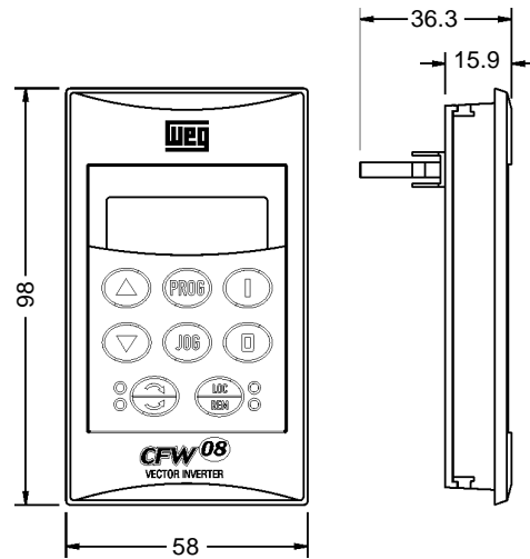
Figura 8.4 -Dimensões da HMI-CFW08-RP
