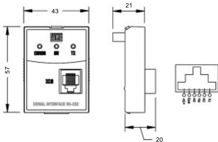
Figura 8.13 - Dimensões do módulo de comunicação serial RS-232 KCS-CFW08 e sinais do conector RJ(XC8)
