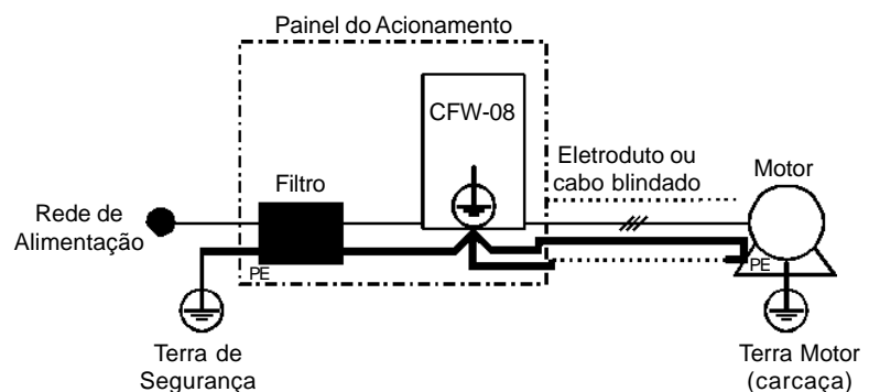
Figura 8.20 - Conexão do filtro supressor de RFI Classe B externo
