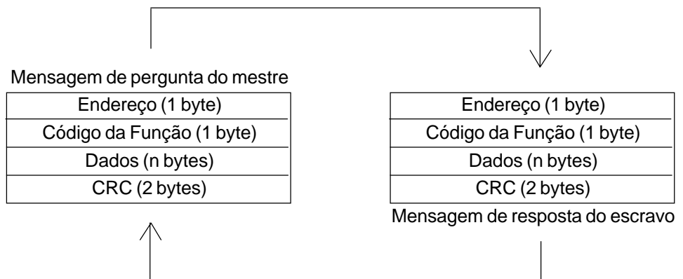
Figura 8.26 - Estrutura das mensagens
