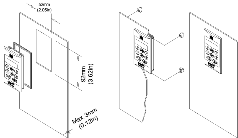
Figura 8.10 - Instalação da HMI-CFW08-RS
