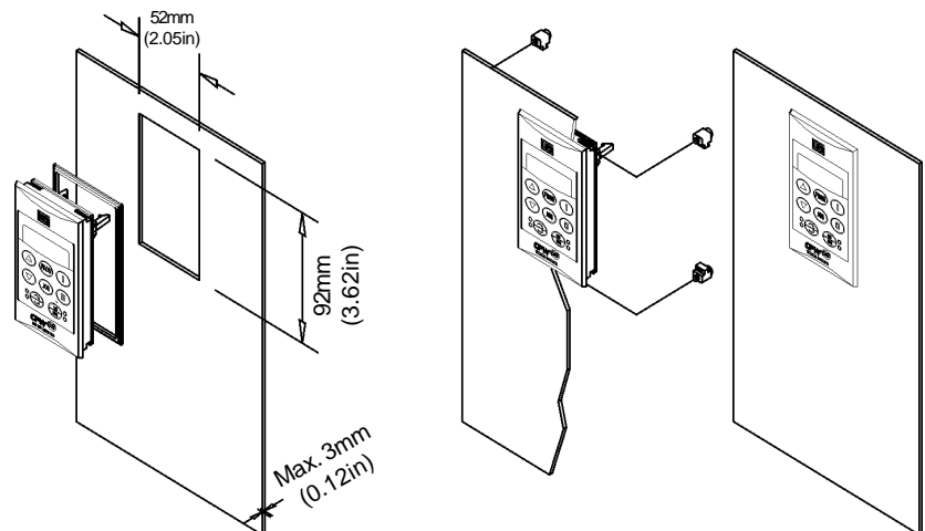
Figura 8.5 -Instalação da HMI-CFW08-RP
