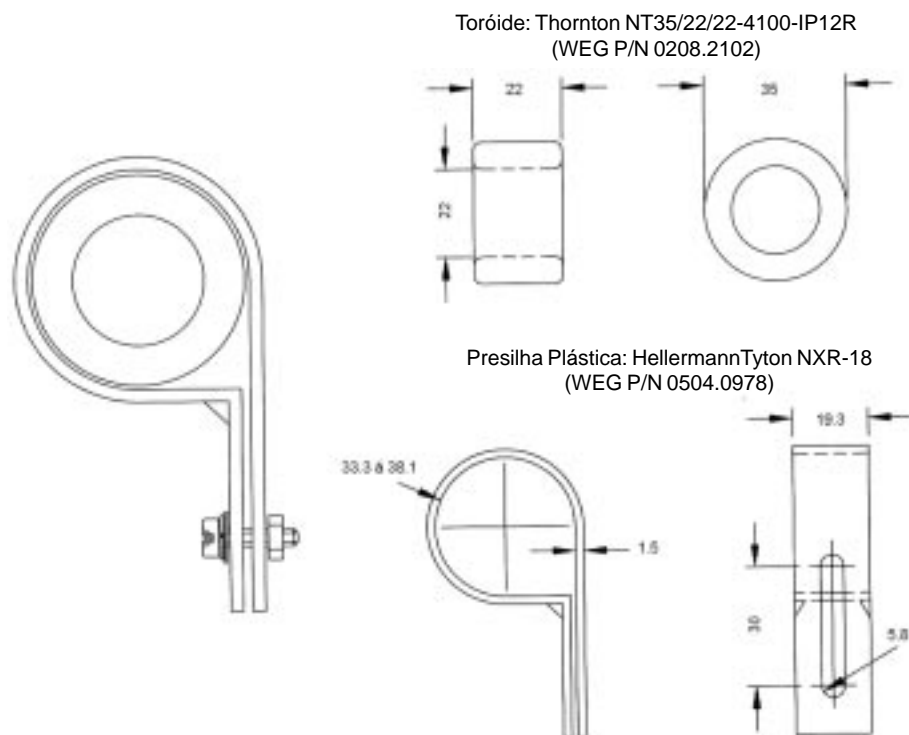
Figura 3.20 - Desenho do kit TOR1-CFW08
