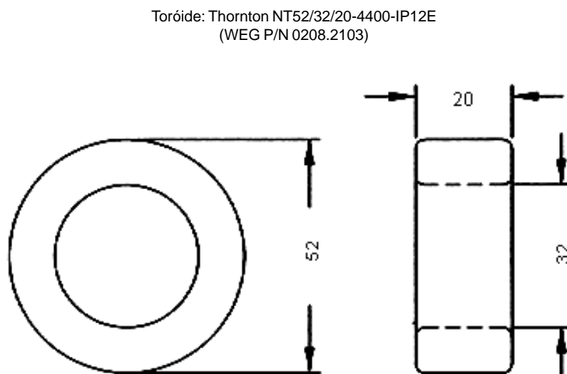
Figura 3.21 - Desenho do toróide TOR2-CFW08
