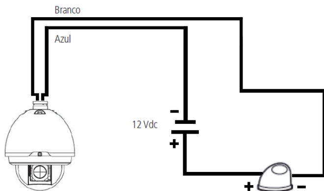
Conexão dos dispositivos de alarme
