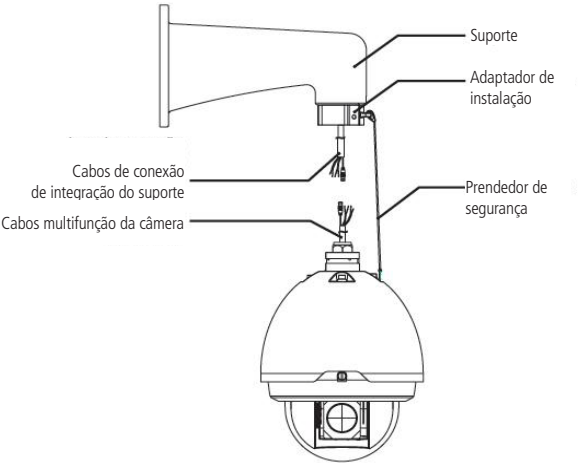
Conexão da speed dome
