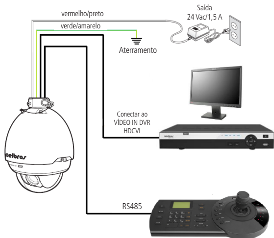
Esquema básico controle HDCVI + RS485
