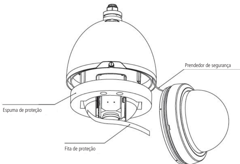
Retirada dos dispositivos de segurança
