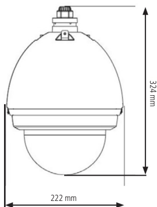
Dimensões da câmera
