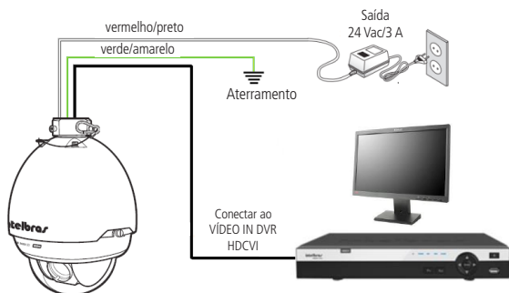
Esquema básico controle HDCVI
