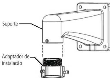
Fixação do adaptador
