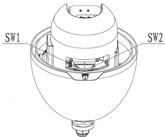
Localização dos dip-switchs
