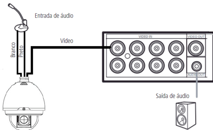
Conexão dos dispositivos de áudio
