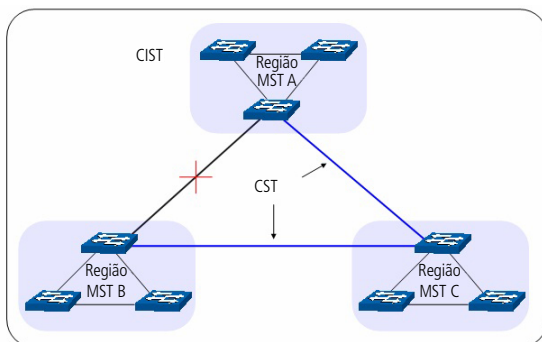
Diagrama de rede MSTP
