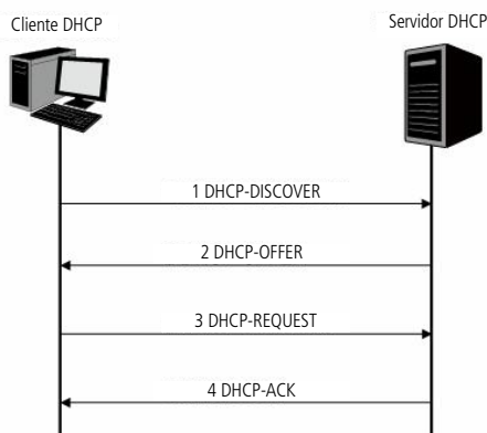
Negociação DHCP
