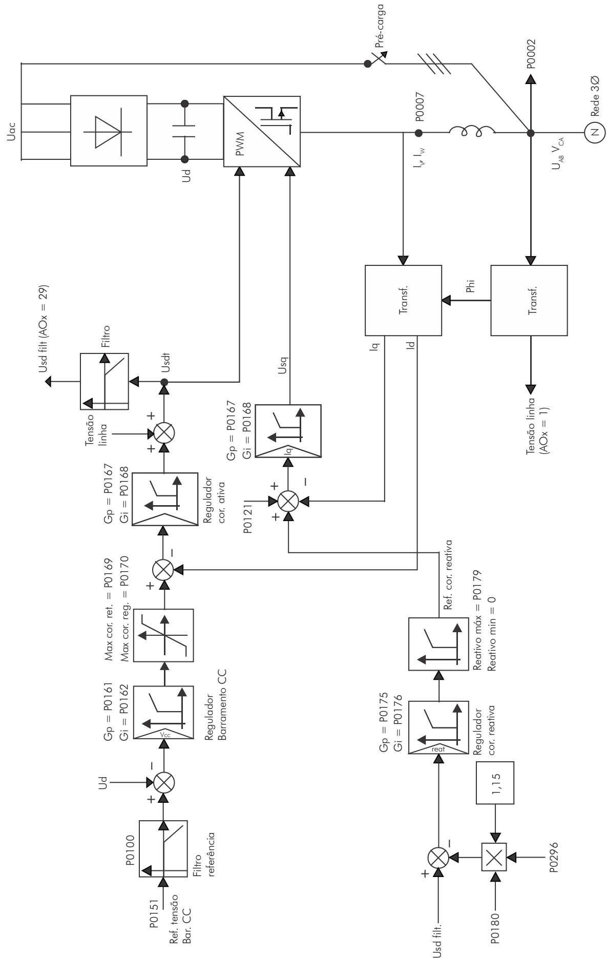
Figura 8.1 - Bloco diagrama do controle vetorial
