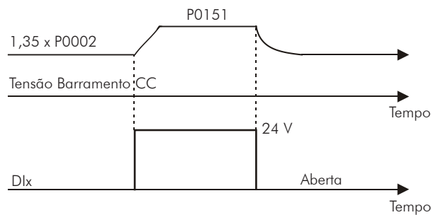
c) RESET
