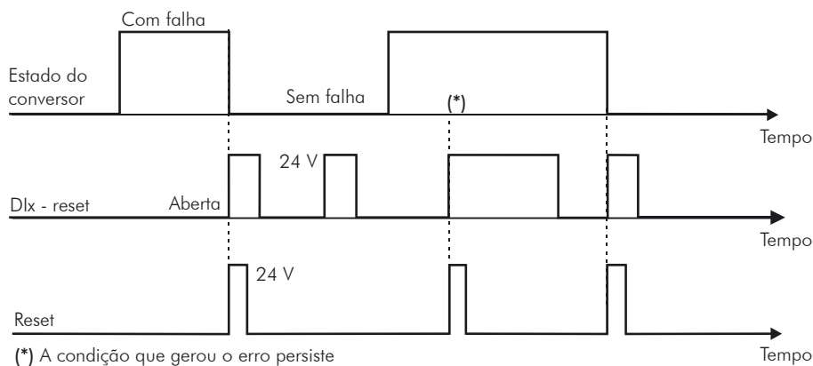
Figura 9.2 - a) a c) Detalhes sobre funcionamento das funções das entradas digitais
