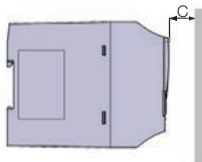
(c) Minimum ventilation free spaces (c) Espacios libres mínimos para ventilación (c) Espaços livres mínimos para ventilação
