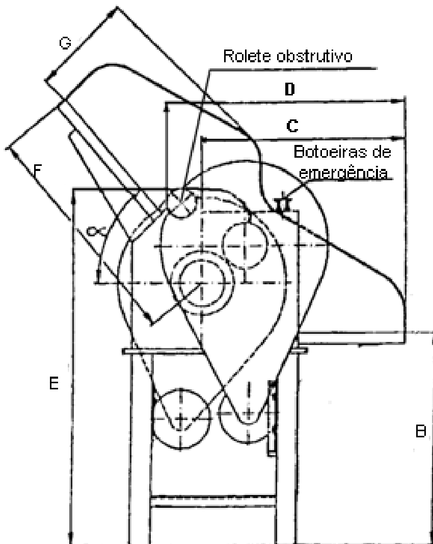
Figura 2: Desenho esquemático do cilindro de panificação.
