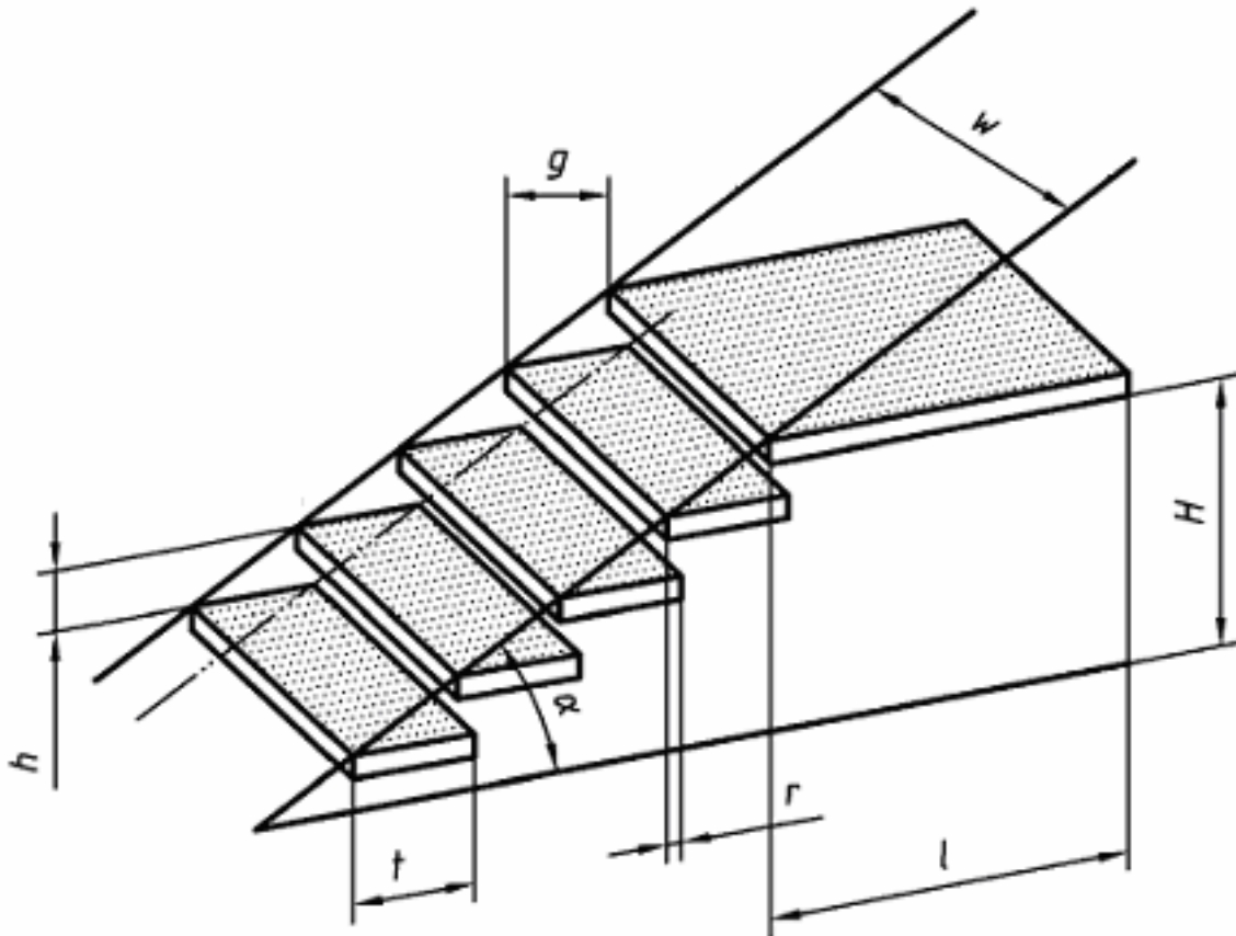
Figura 2: Exemplo de escada sem espelho.
