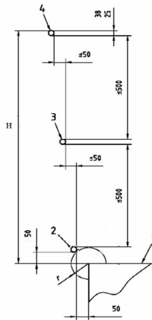
Figura 5: Sistema de proteção contra quedas em plataforma de trabalho com acúmulo de sujidades. (dimensões em milímetros)
