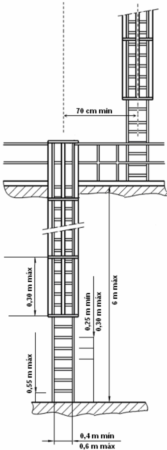
Figura 3: Exemplo de escada fixa do tipo marinheiro.
