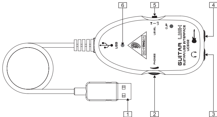
Fig. 2.1: Componentes e ligações
