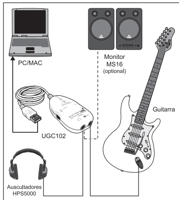
Fig. 4.1: Cablagem da UCG102
