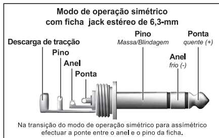
Fig. 5.2: jaque estéreo de 6,3 mm
