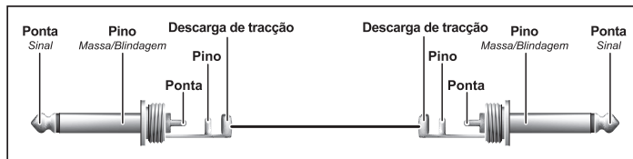
Fig. 5.1: A instalação de um cabo mono jaque
