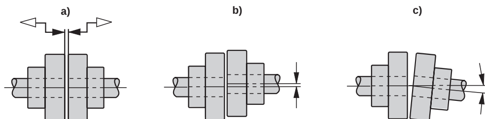
Figura 6: Folga e desalinhamento para instalação de acoplamentos
