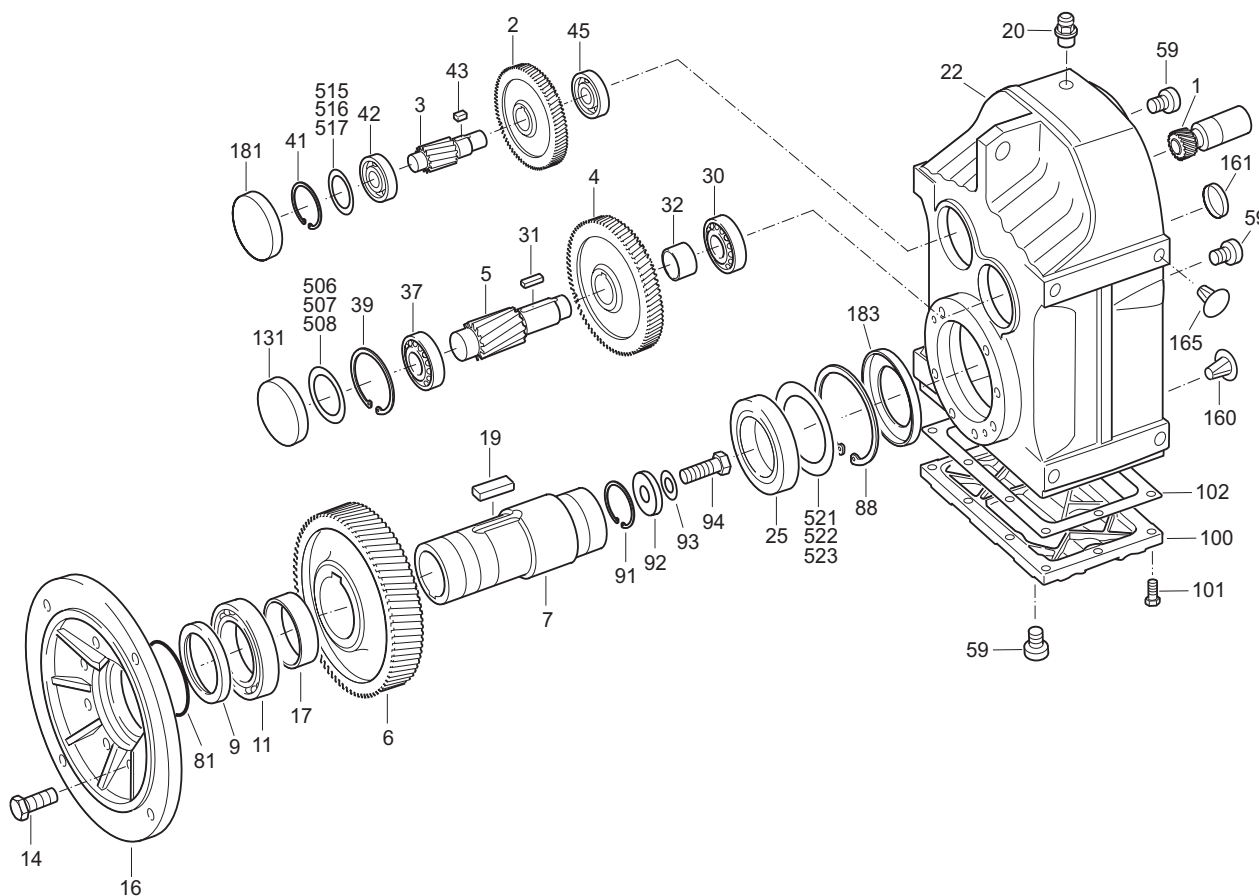
Figura 2: Estrutura geral do redutor helicoidal de veios paralelos
