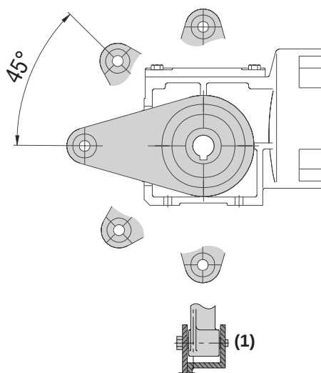
Figura 10: Braço de binário para redutores SPIROPLAN® W
