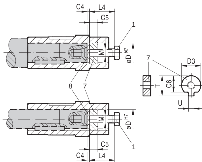
Figura 11: Kit de montagem/desmontagem SEW-EURODRIVE
