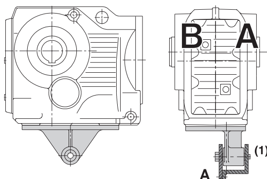
Figura 8: Braço de binário para redutores cónicos
