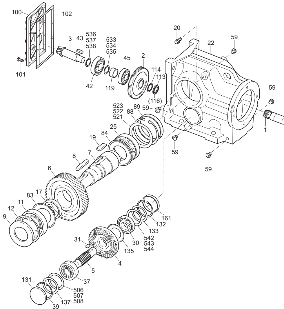
Figura 3: Estrutura geral do redutor cónico
