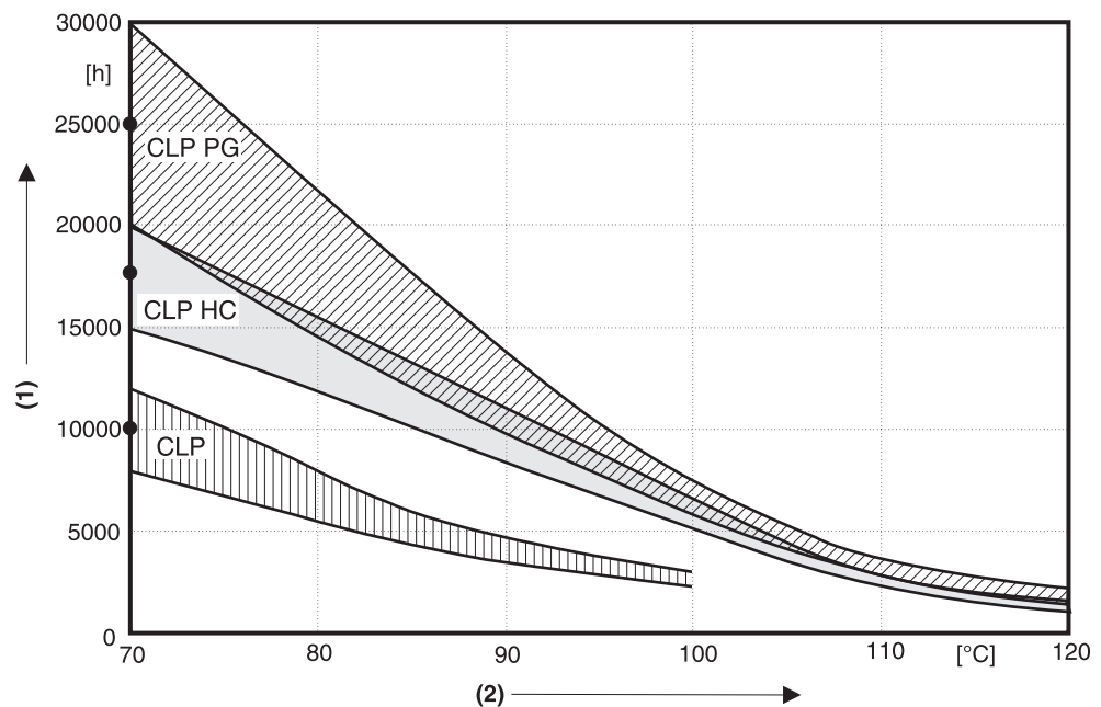
Figura 12: Intervalos de substituição de óleo para redutores standard em condições ambientais normais..
