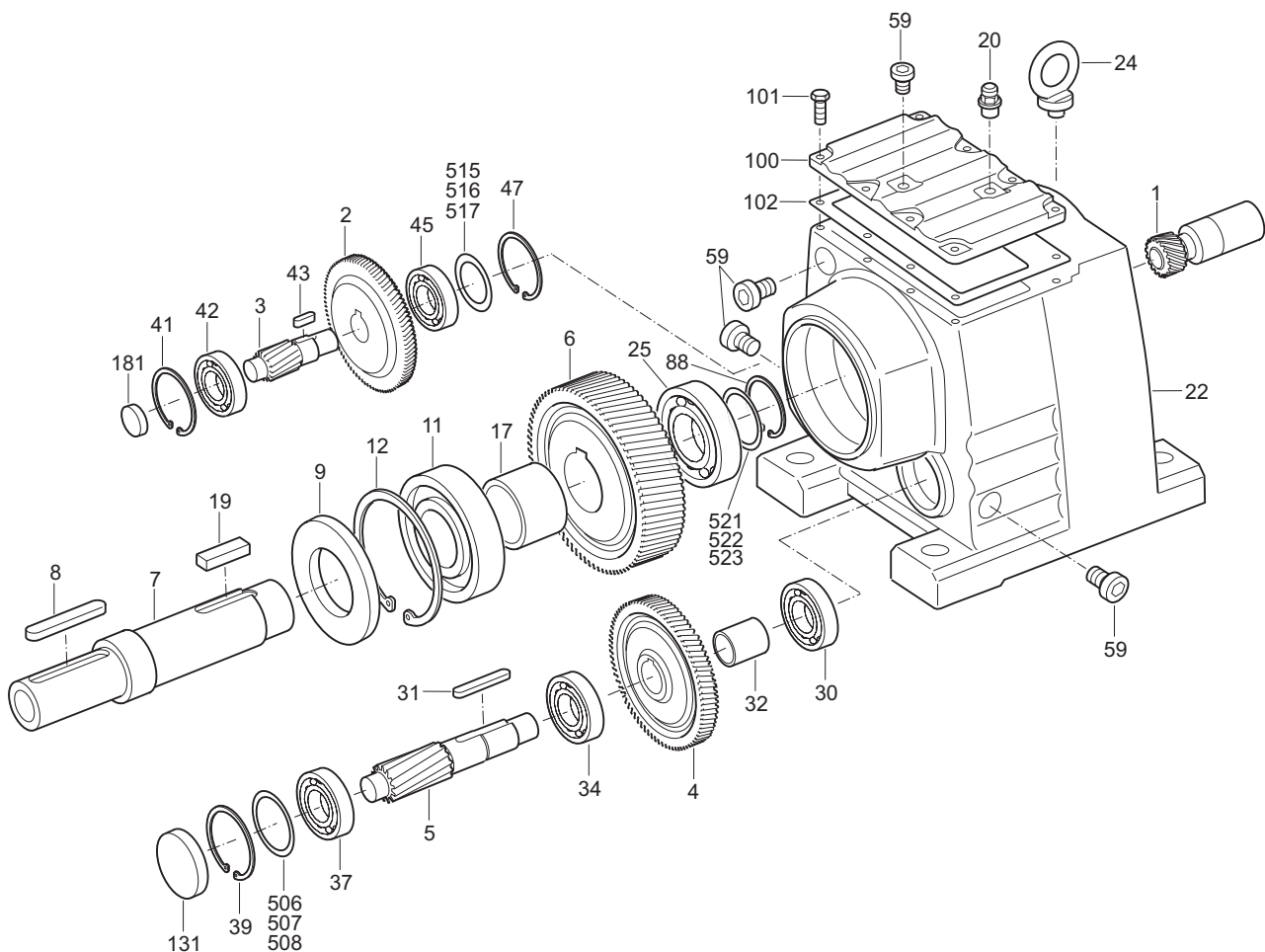
Figura 1: Estrutura geral do redutor helicoidal
