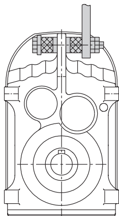
Figura 7: Braço de binário para redutores de veios paralelos
