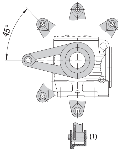
Figura 9: Braço de binário para redutores sem-fim
