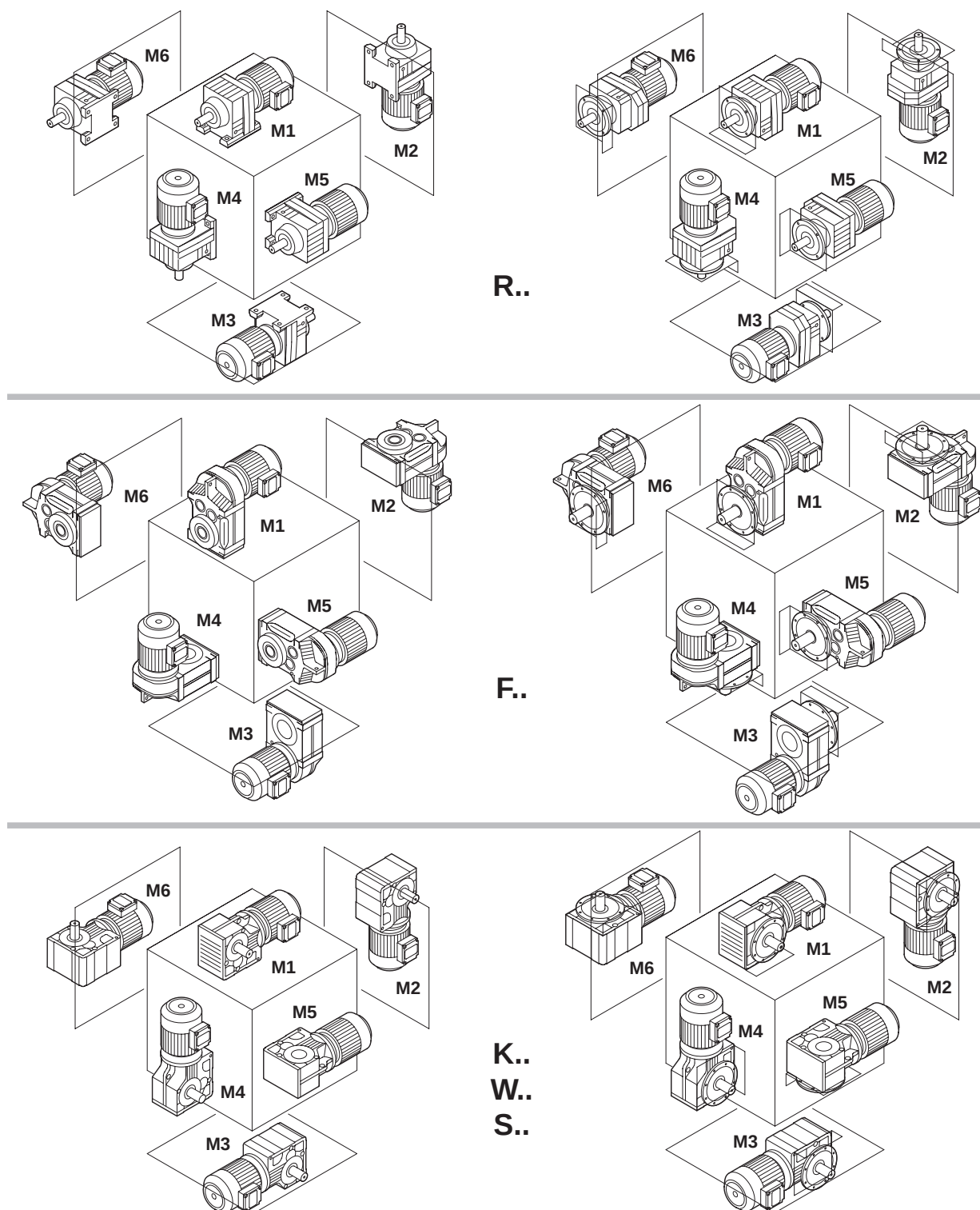
Figura 13: Posições de montagem M1 M6
