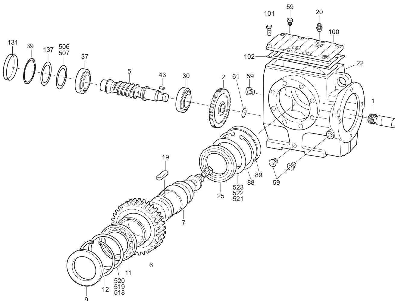
Figura 4: Estrutura geral do redutor sem-fim
