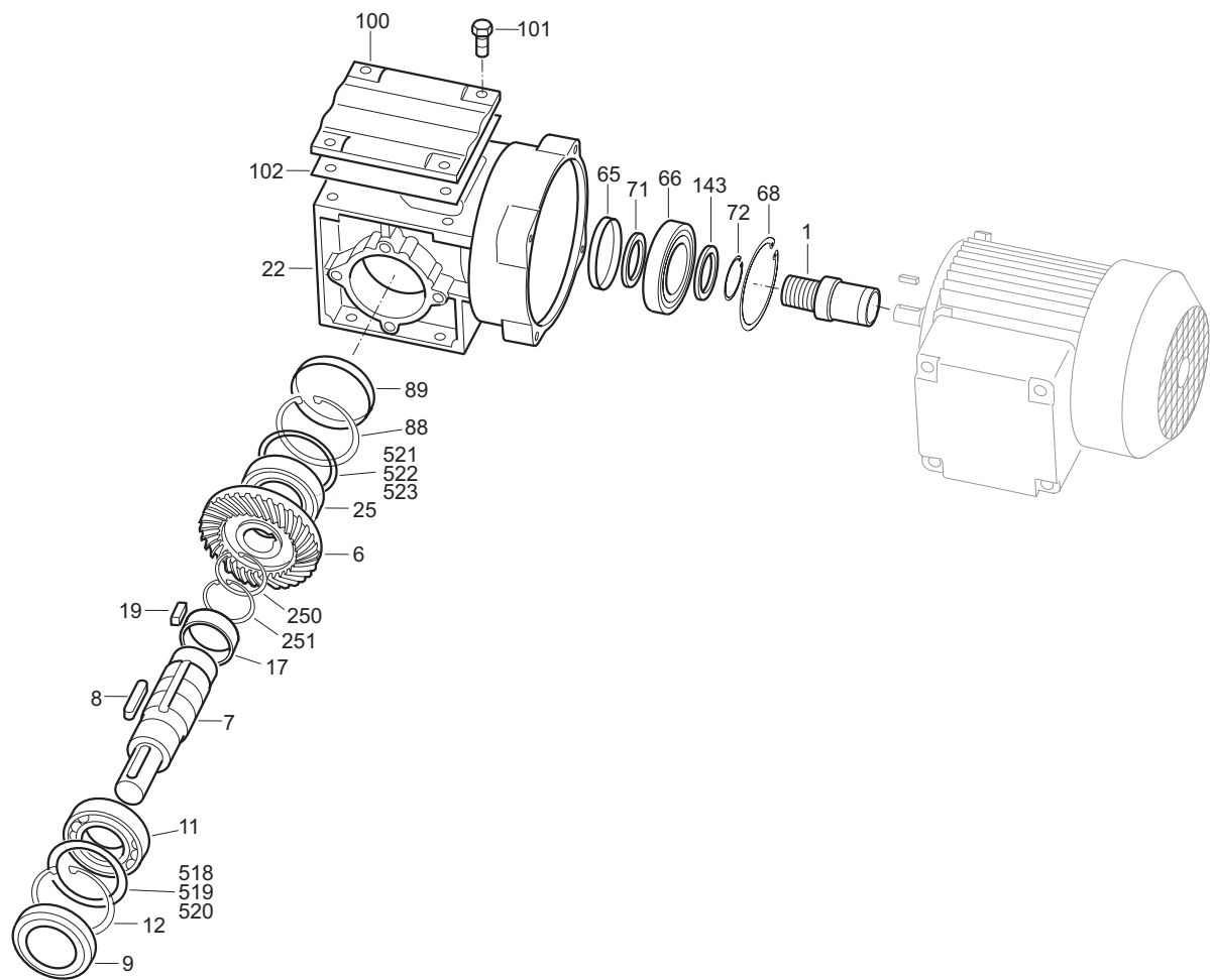
Figura 5: Estrutura geral do redutor SPIROPLAN®
