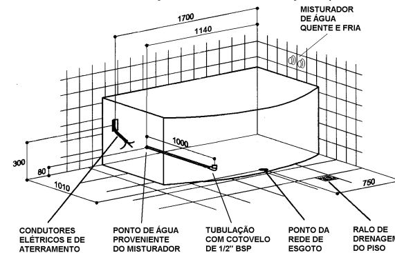
REQUISITOS PARA INSTALAÇÃO - MOTOBOMBA POSIÇÃO 2 (LADO ESQUERDO)
