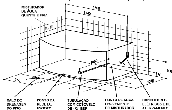
REQUISITOS PARA INSTALAÇÃO - MOTOBOMBA POSIÇÃO 1 (LADO DIREITO)
