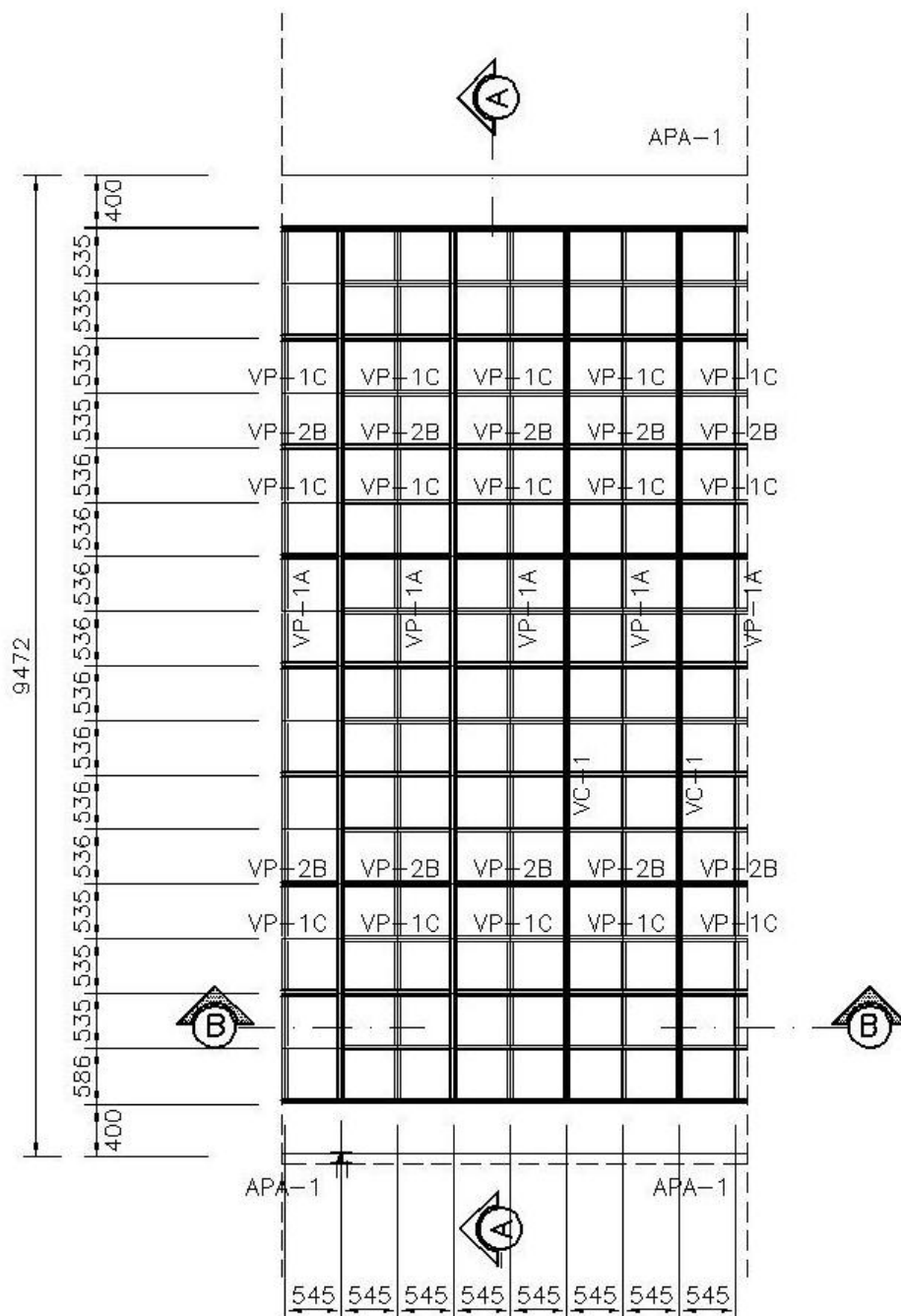
PLANTA BAIXA: PERGOLADO (parcial)
