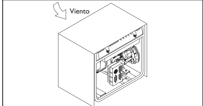
Figura 12 — Refugio Frío Permanente del Tiempo
