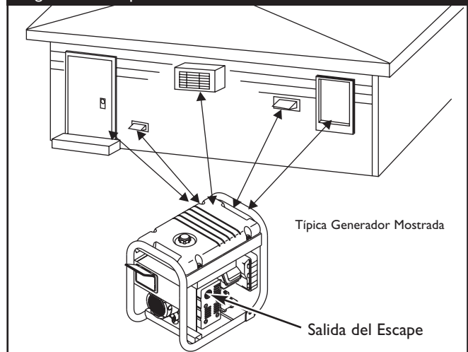
Figura 10 — Espacio Libre Alrededor del Generador
