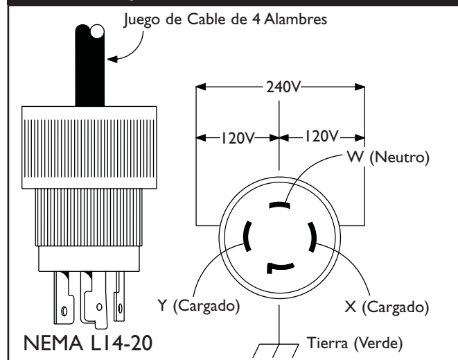
Figura 13 — 120/240 Volt AC, 20 Amperios, Receptáculo de Seguridad
