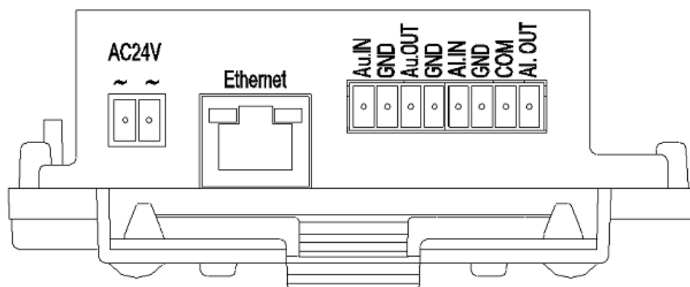
FIGURA 1-4: DEFINIÇÕES DE PIN 2/2
