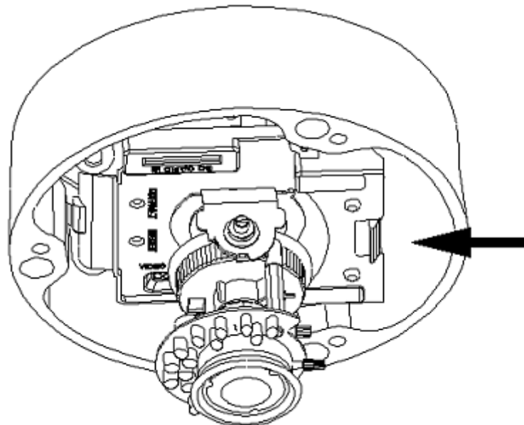
FIGURA 2-3: CONEXÃO DOS FIOS
