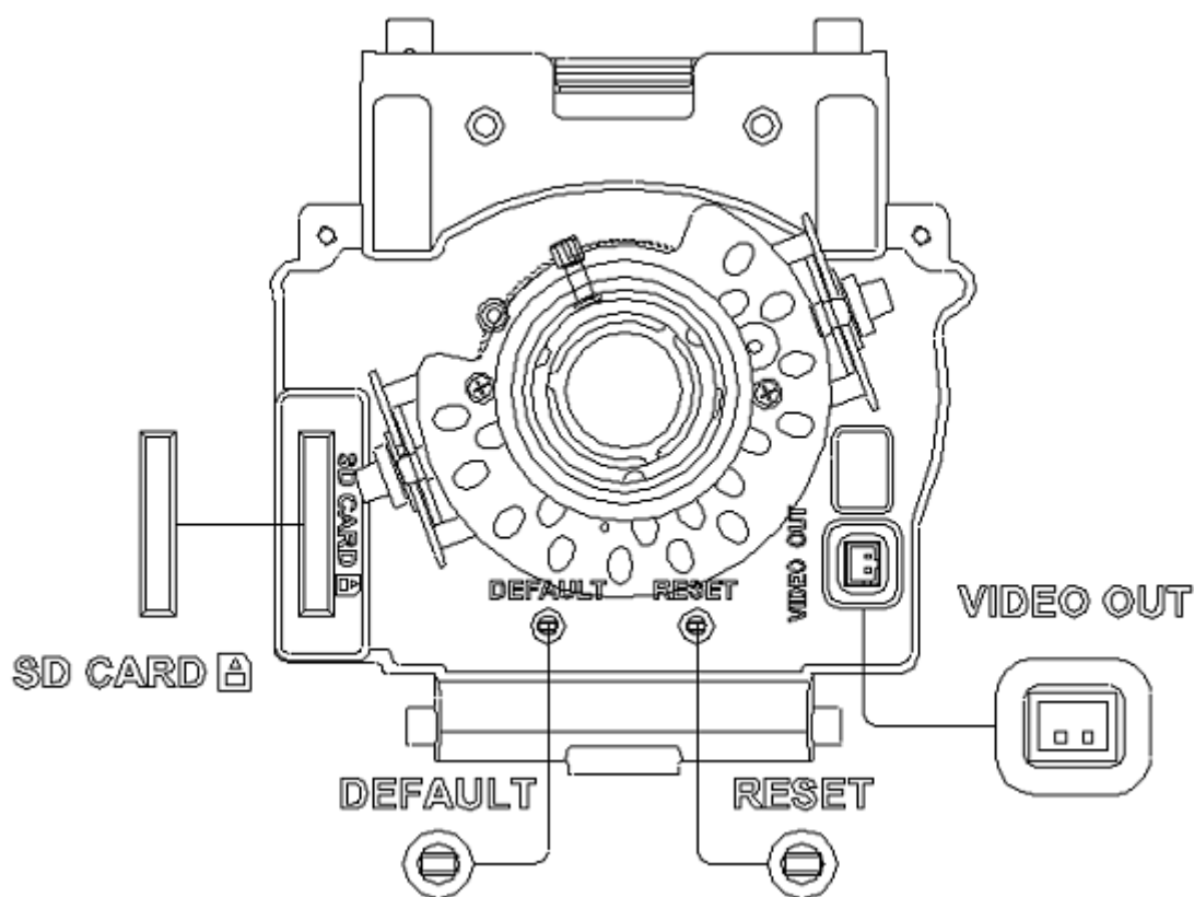
FIGURA 1-3: DEFINIÇÕES DE PIN 1/2
