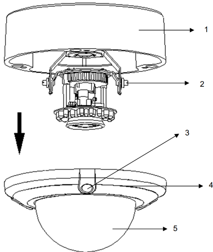
FIGURA 2-1: DESMONTAGEM DA CÂMERA
