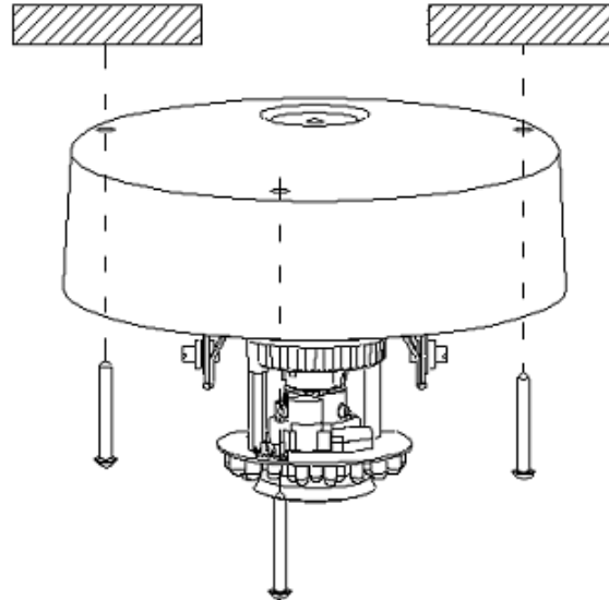
FIGURA 2-4: MONTAGEM DA CÂMERA
