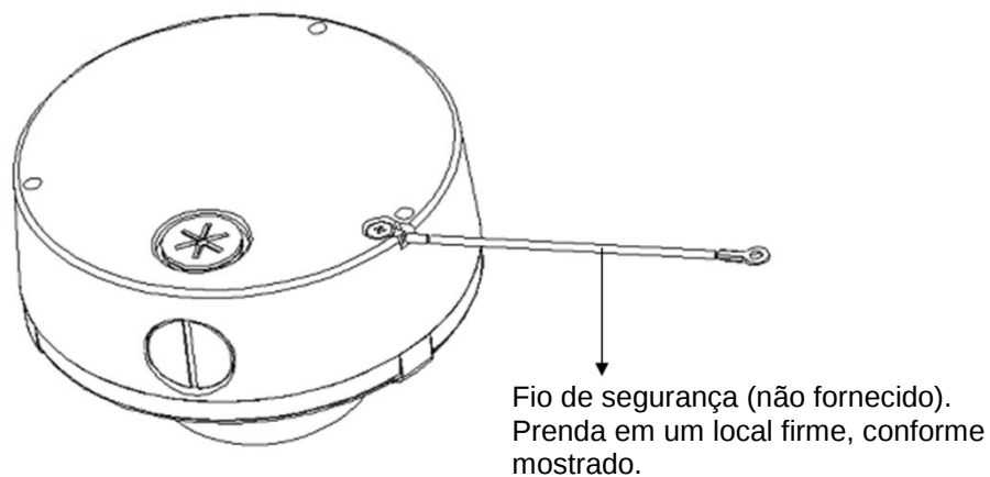
FIGURA 2-5: MONTAGEM DA CÂMERA
