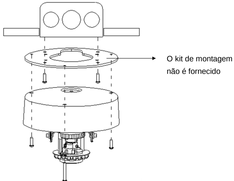
FIGURA 2-6: MONTAGEM DA CÂMERA
