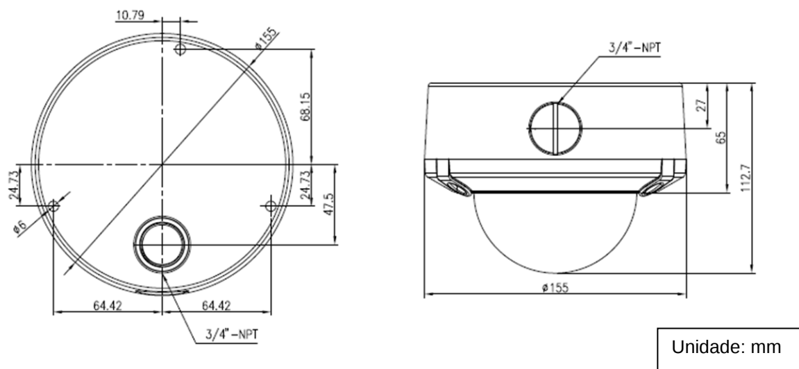
FIGURA 1-1: DIMENSÃO FÍSICA A
