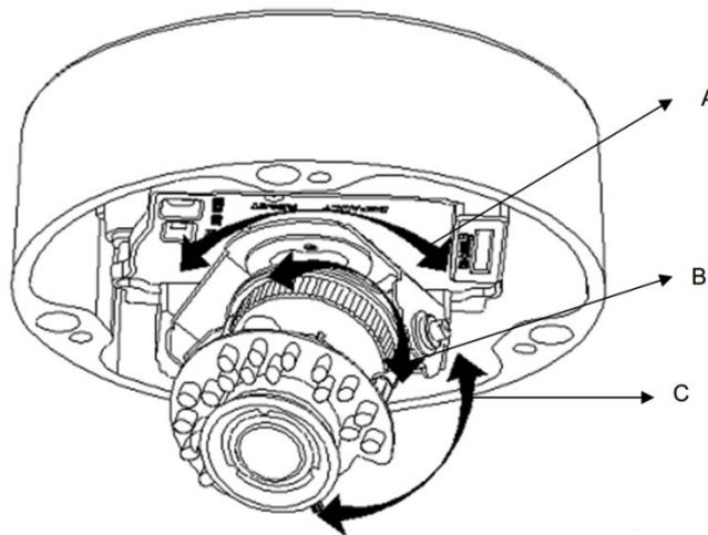
FIGURA 2-7: AJUSTE DA POSIÇÃO DA CÂMERA
