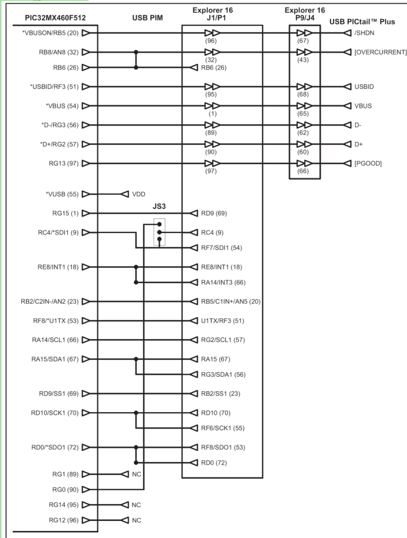
Figura 4.1 – Pinos roteados no plugin
