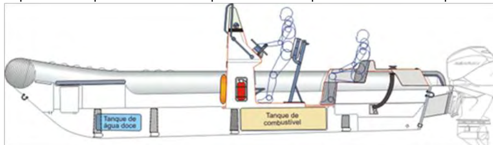
Motor de popa
