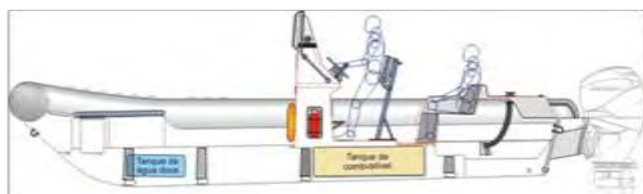
Lazer Standard console tipo militar
