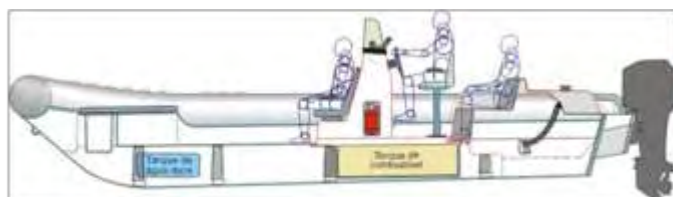
Lazer Standard console tipo Tour
