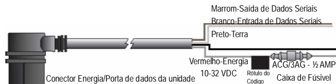
Cabo Energia/Dados de porta serial com terminal de arame opcional
