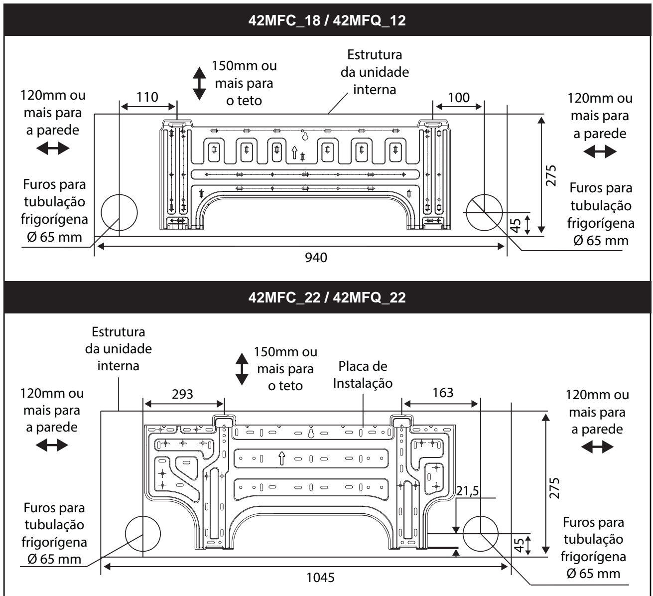
FIG. 20-B - PLACAS DE MONTAGEM
