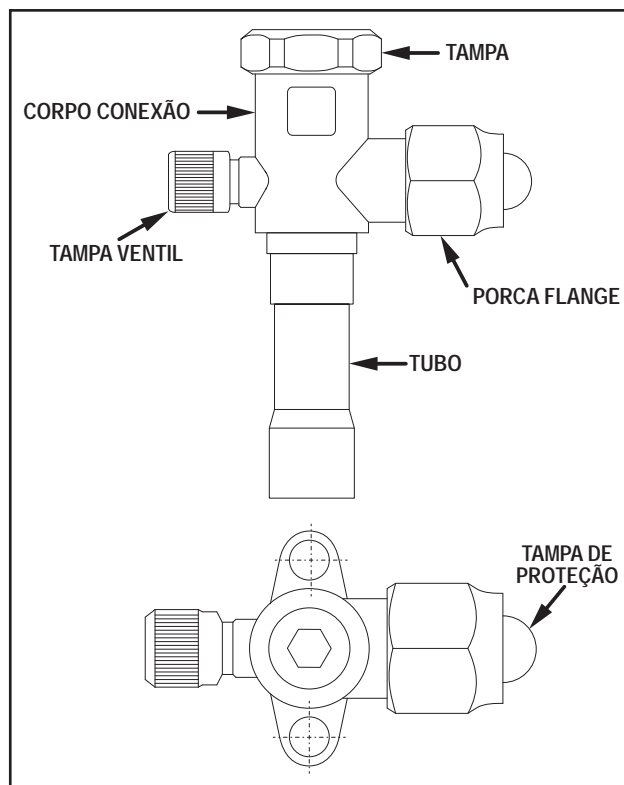
FIG. 24 - VÁLVULA DE SERVIÇO LINHAS SUÇÇÃO/EXPANSÃO
