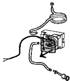
1) Retirar a tampa transparente
