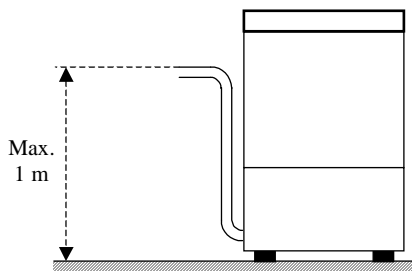
Com bomba de escoamento ( disponível a pedido )
