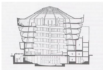
Figura 12: Museu Guggenheim, Nova York. Corte transversal. Fonte: Montaner
