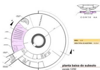
Figura 34.: MAC, Niterói. Planta baixa subsolo. Fonte: www.macniteroi.com.br
