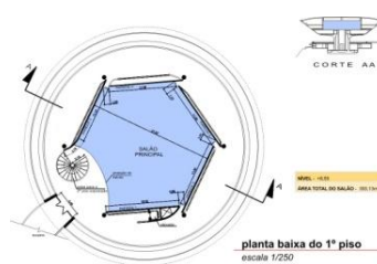
Figura 35: MAC, Niterói. Planta baixa do 1º piso. Fonte: www.macniteroi.com.br
