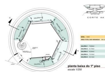
Figura 36: MAC, Niterói. Planta baixa do 1º piso. Fonte: www.macniteroi.com.br
