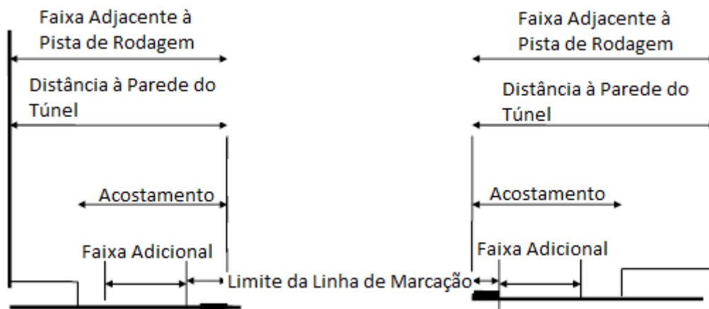
Figura 4.3 – Elementos da área adjacente à pista de rodagem (PIARC, 2001).
