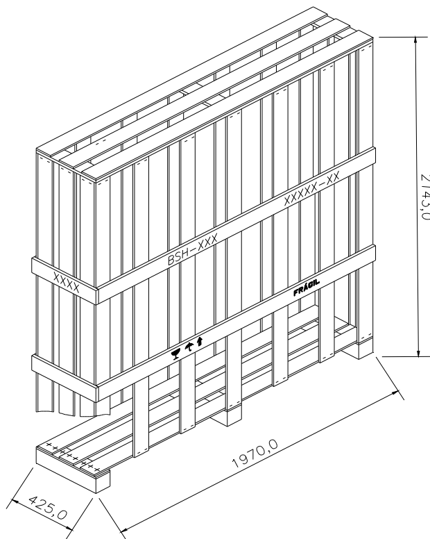
FIGURA 02 – Embalagem do refletor
