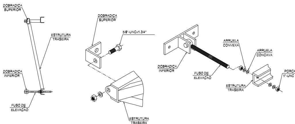
FIGURA 07 – Montagem da estrutura traseira
