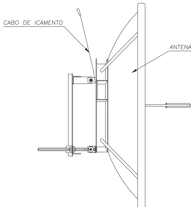
FIGURA 11 - Içamento
