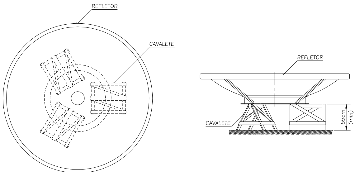
FIGURA 06 – Apoio para o refletor
