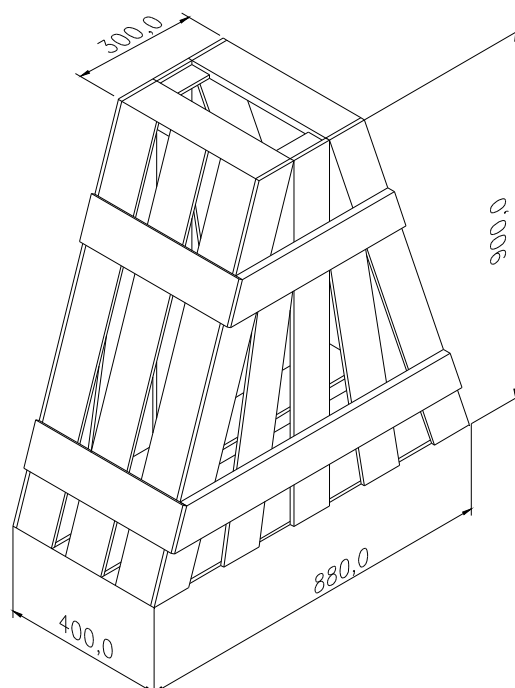
FIGURA 04 – Embalagem da estrutura traseira
