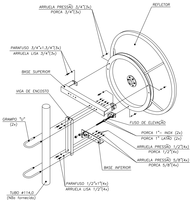
FIGURA 12 – Fixação no tubo suporte
