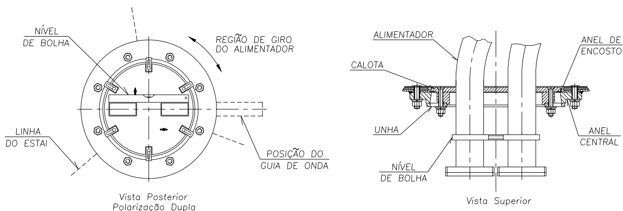
FIGURA 13 – Alimentador/polarização
