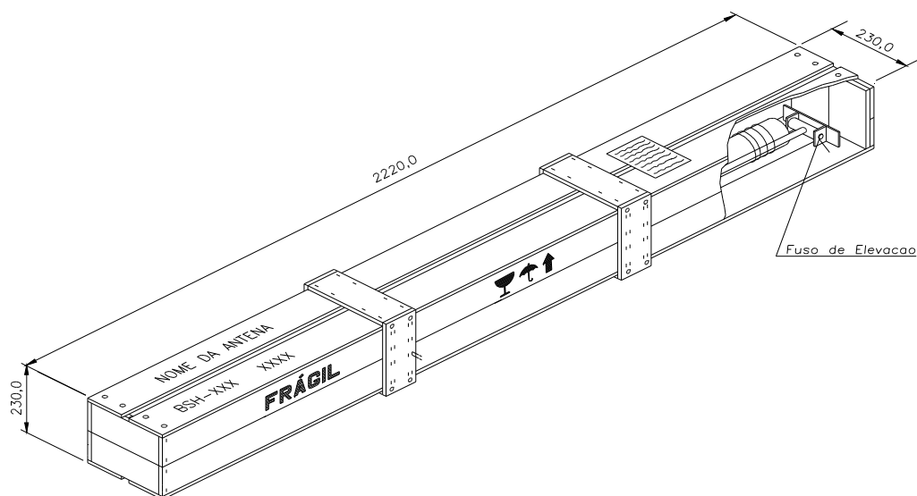
FIGURA 05 – Embalagem das barras estabilizadoras
