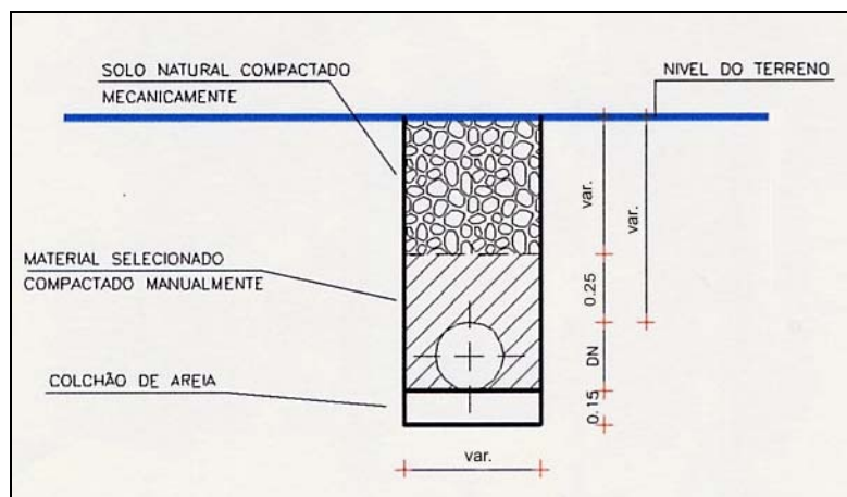
Figura 1 - Esquema de valas e assentamento de tubos.
