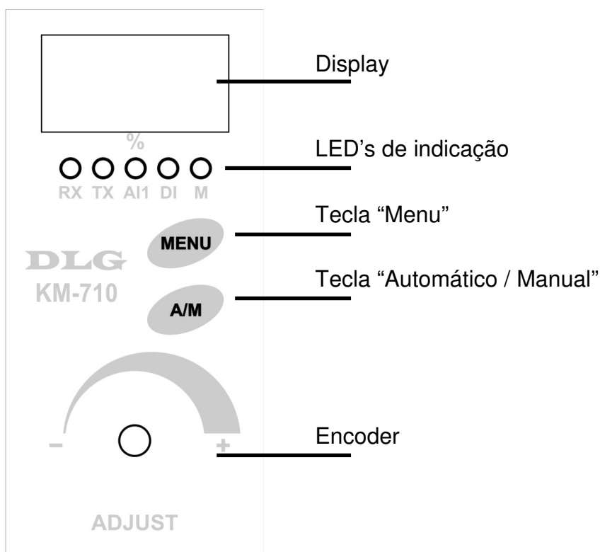
Figura 1 Painel Frontal da KM-710
