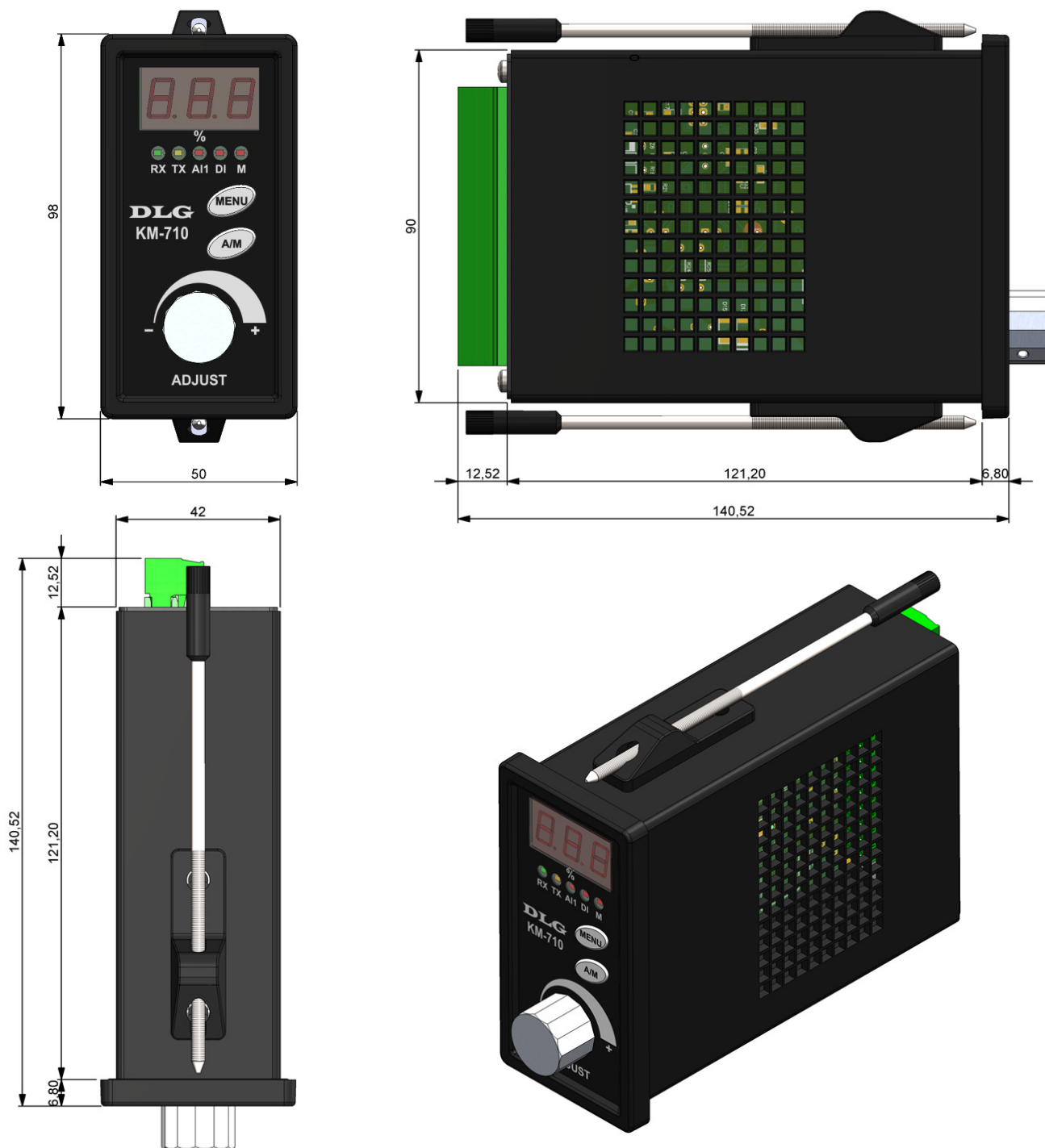
Figura 2 Dimensionamento (Cotas em milímetro)
