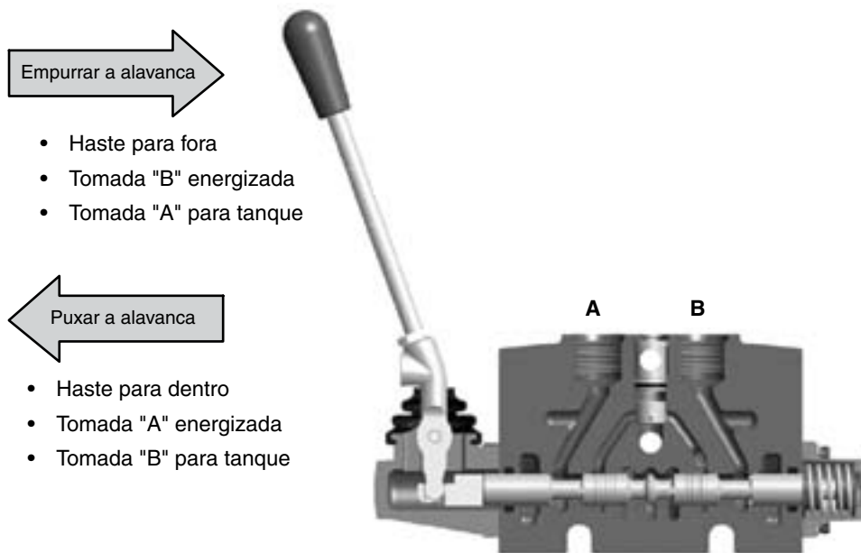
Figura 13 - Vista a montante
