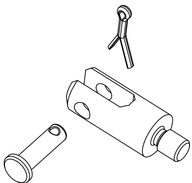
Figura 15a Extensão fêmea Conjunto 1715019 Torque = 2 – 3 N.m ( 18 – 25 Lbf.pé) Aplique trava-rosca antes da montagem
