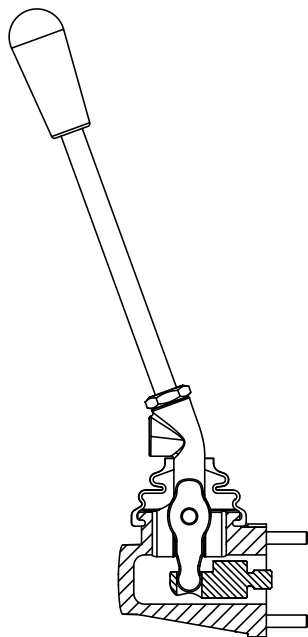
Figura 15 Conjunto alavanca
