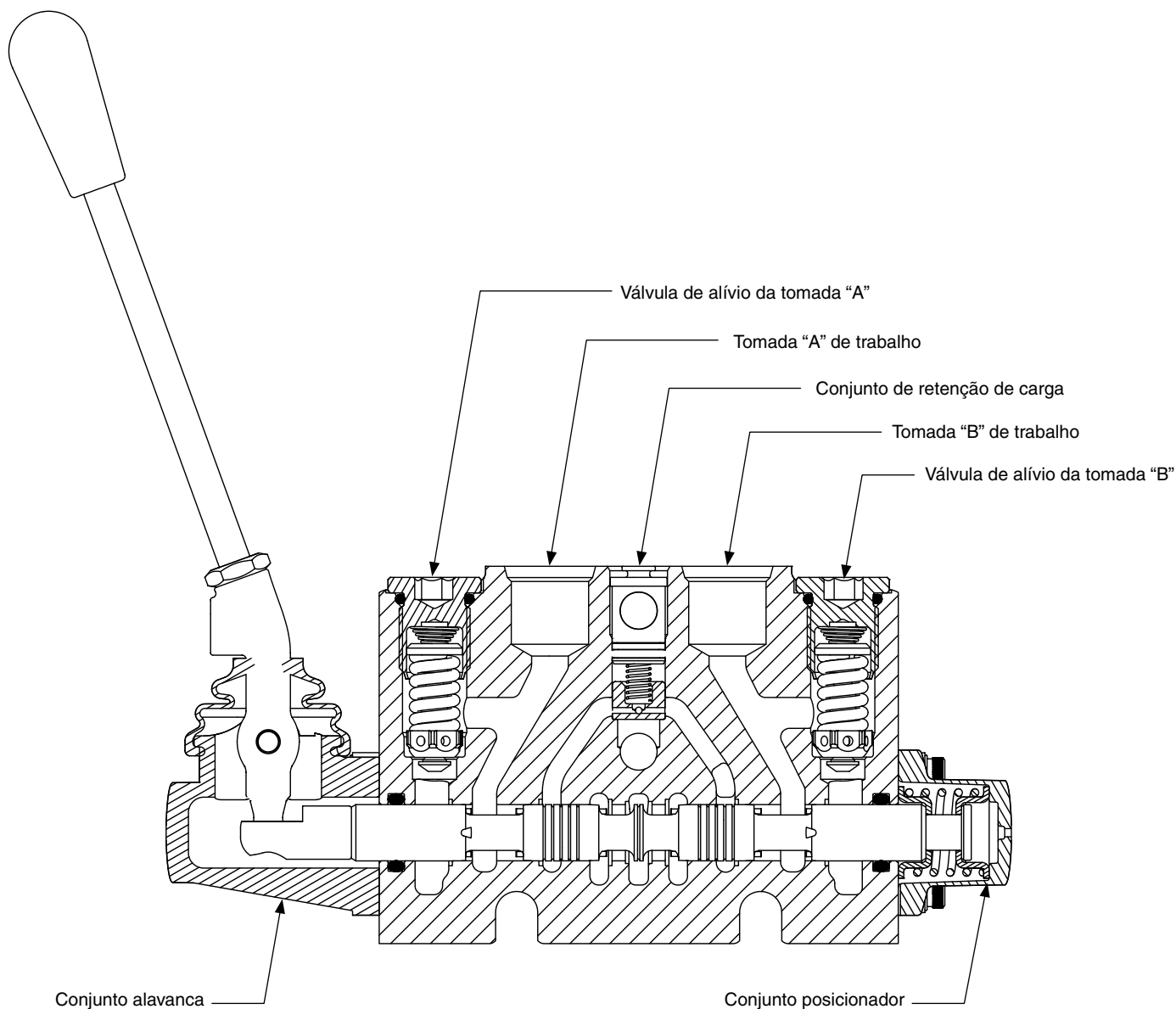
Figura 1 - Vista montante
