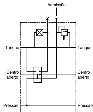
Combinadora de vazão
