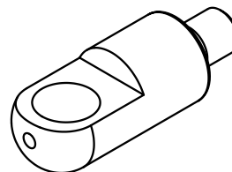
Figura 15b Extensão da haste (Para ser utilizado nos conjuntos 1715018 e 1715038) Torque = 2 – 3 N.m ( 18 – 25 Lbf.pé) Aplique trava-rosca antes da montagem
