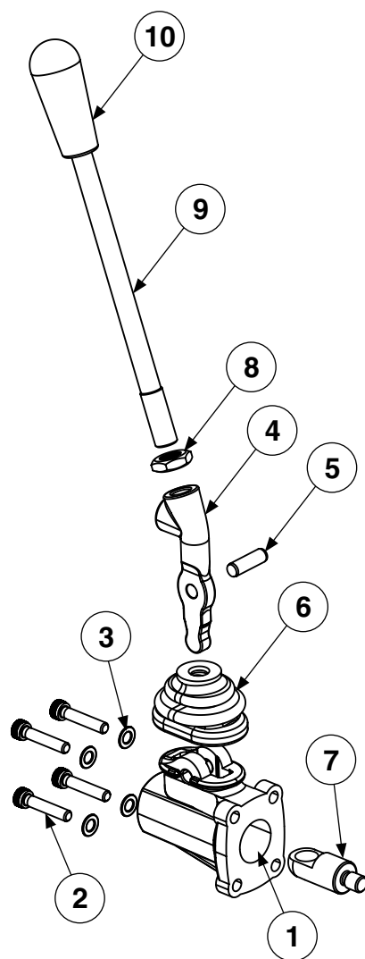
Figura 16 Componentes do conjunto alavanca
