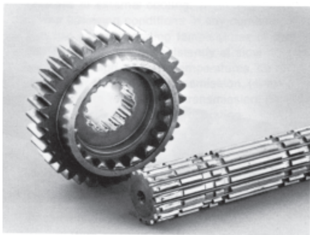
Estriados corroídos
