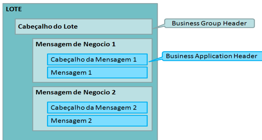
Estrutura de um Arquivo de Negócio.
