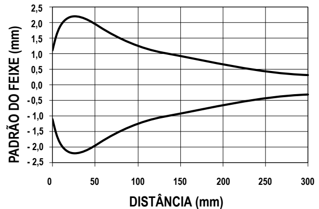
Figura 7: Padrão do Feixe
