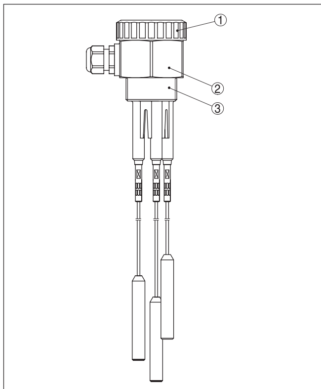
Fig. 1: Sonda condutiva de medição com vários cabos de aço EL 6
