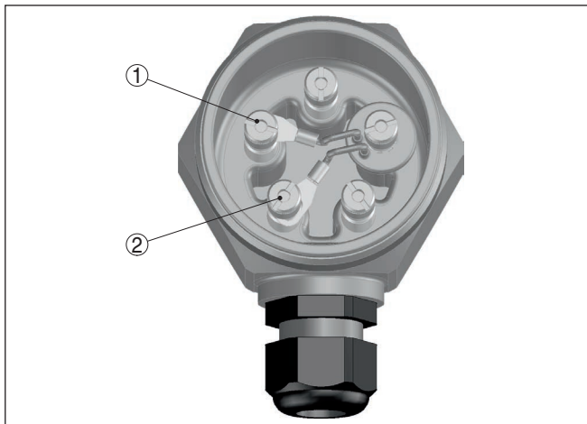
Fig. 6: Montagem do sistema eletrônico adicional para a monitoração do cabo
