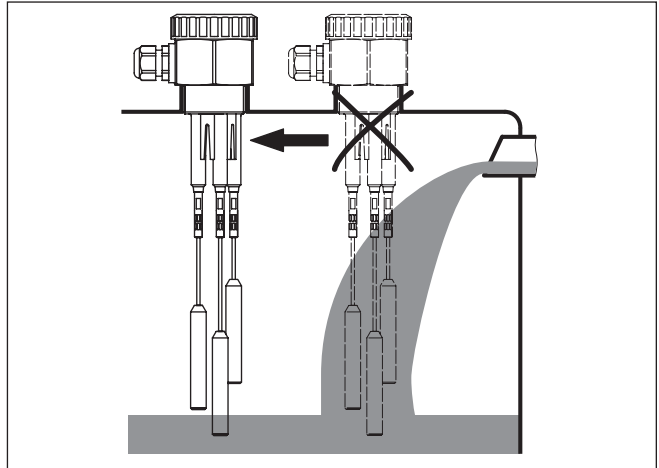
Fig. 3: Fluxo de entrada do produto
