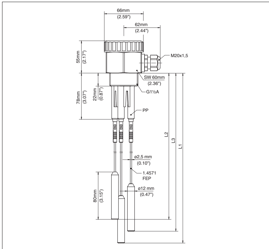
Fig. 7: Sonda condutiva de medição com vários cabos de aço EL 6
