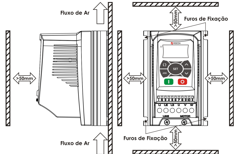
Figura 6-1 – Fixação do Inversor
