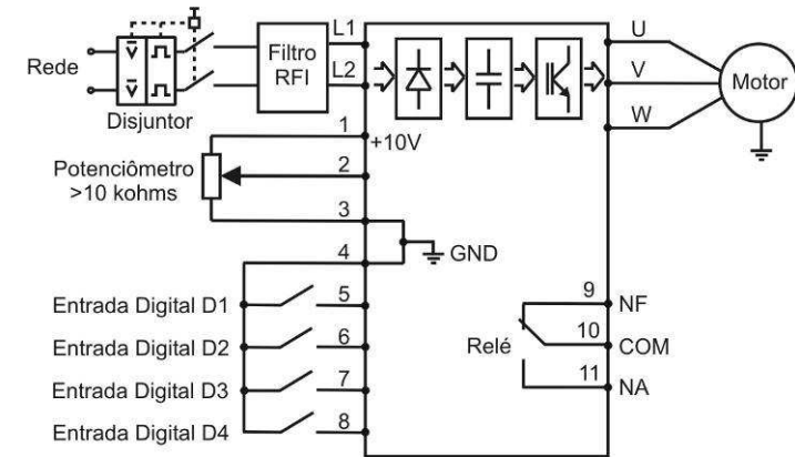
Figura 10-4 – Esquema Elétrico Resumido
