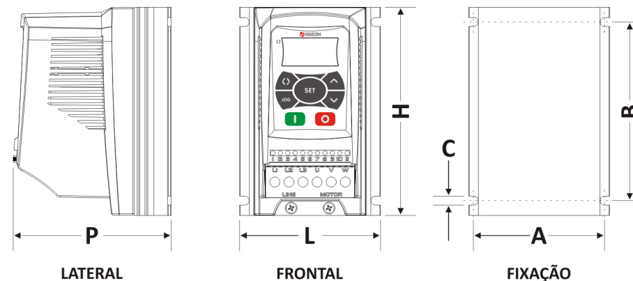
Figura 16-1 – Dimensões
