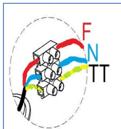
Figura 3 (Conexão elétrica)
