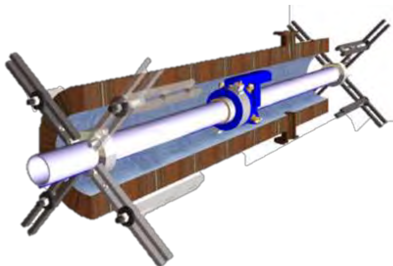
Maquinagem de molde com comprimento de 5600mm e diâmetro de 600mm.
