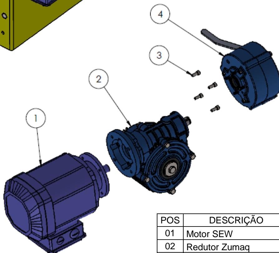
Motor – Redutor – Freio Eletromagnético
