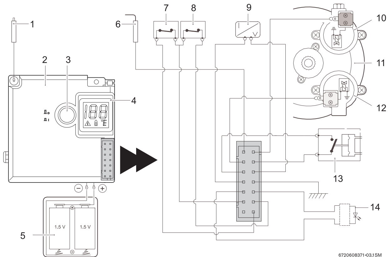
Fig. 3 Esquema elétrico
