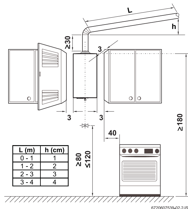
Fig. 4 Distâncias mínimas
