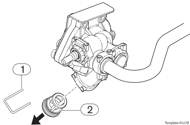
Fig. 16 Purga
