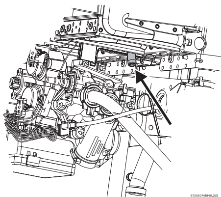
Fig. 14 Ponto de medição de pressão
