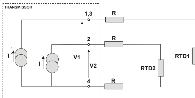
Figura 2.6 - Conexão Diferencial
