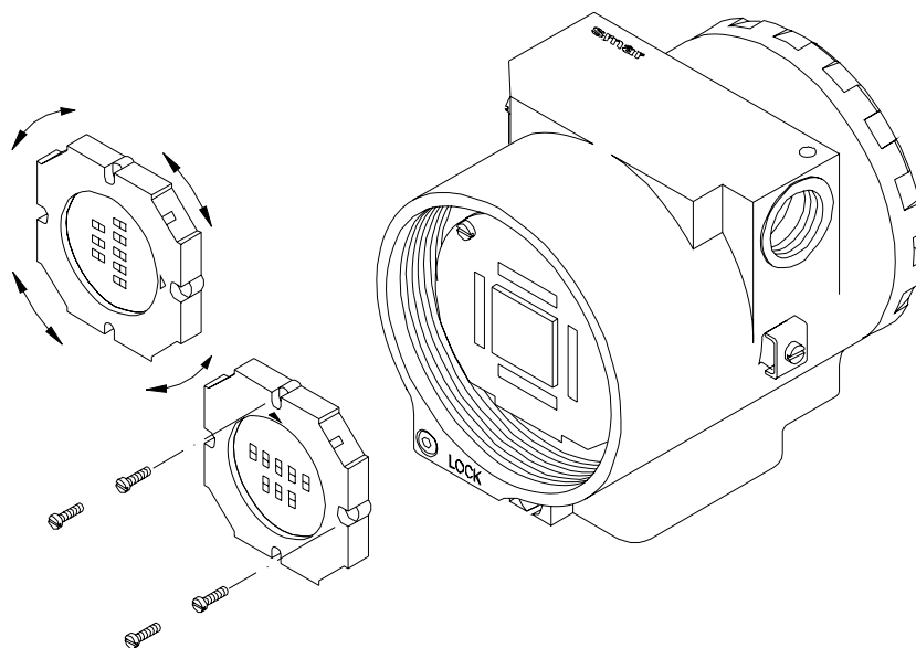
Figura 5.2 – Quatro Posições Possíveis do Display
