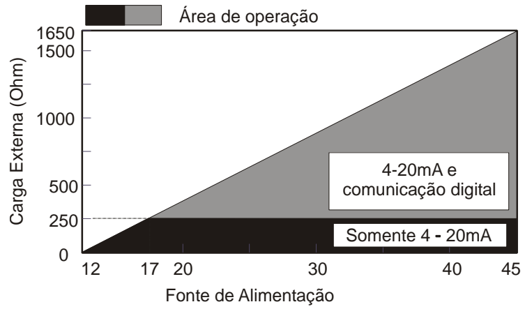
Figura 1.9 - Retas de Carga
