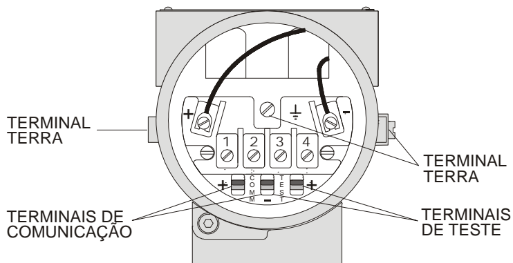
Figura 1.5 - Terminais de Terra
