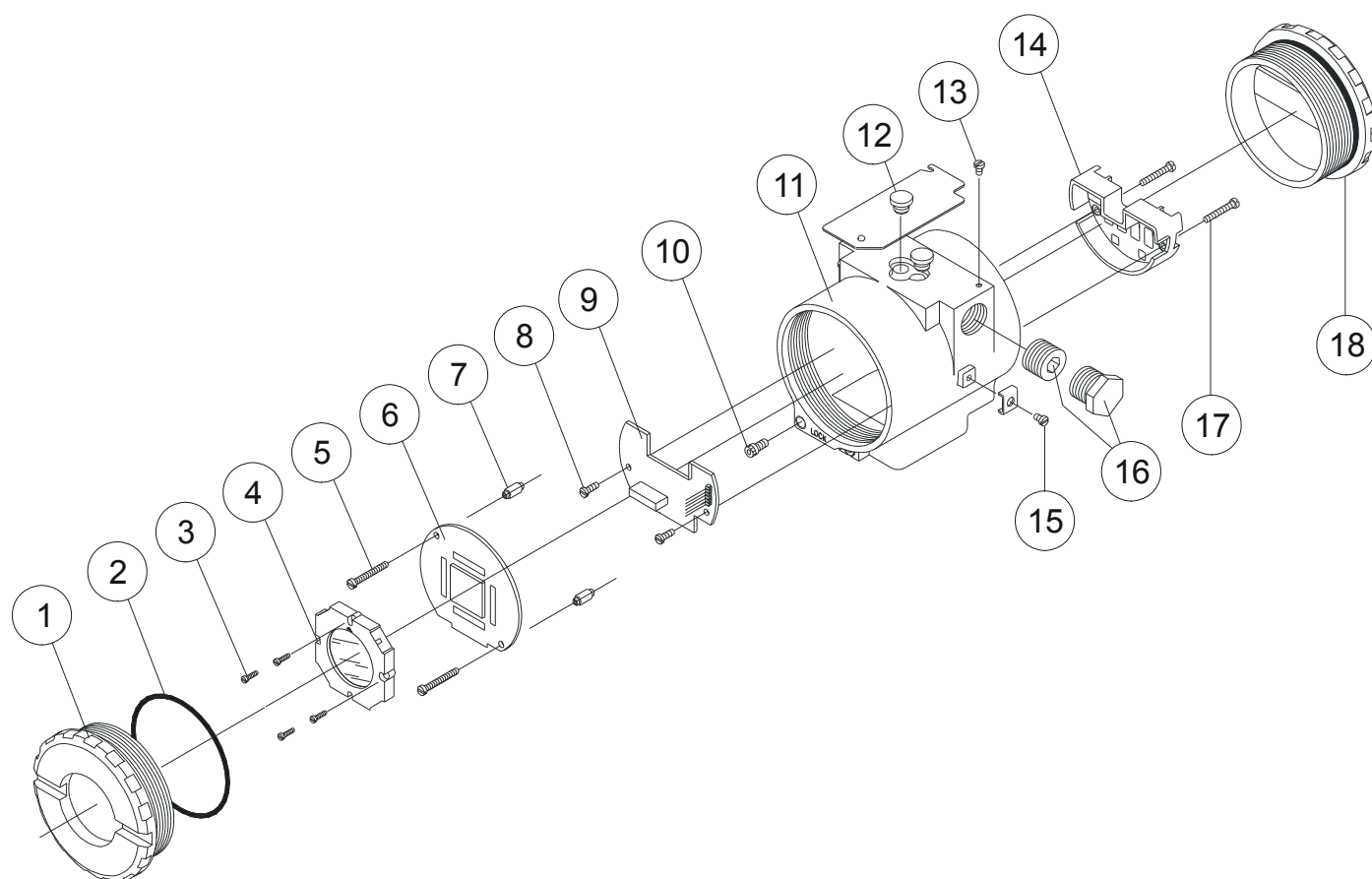
Figura 5.1 – Desenho Explodido
