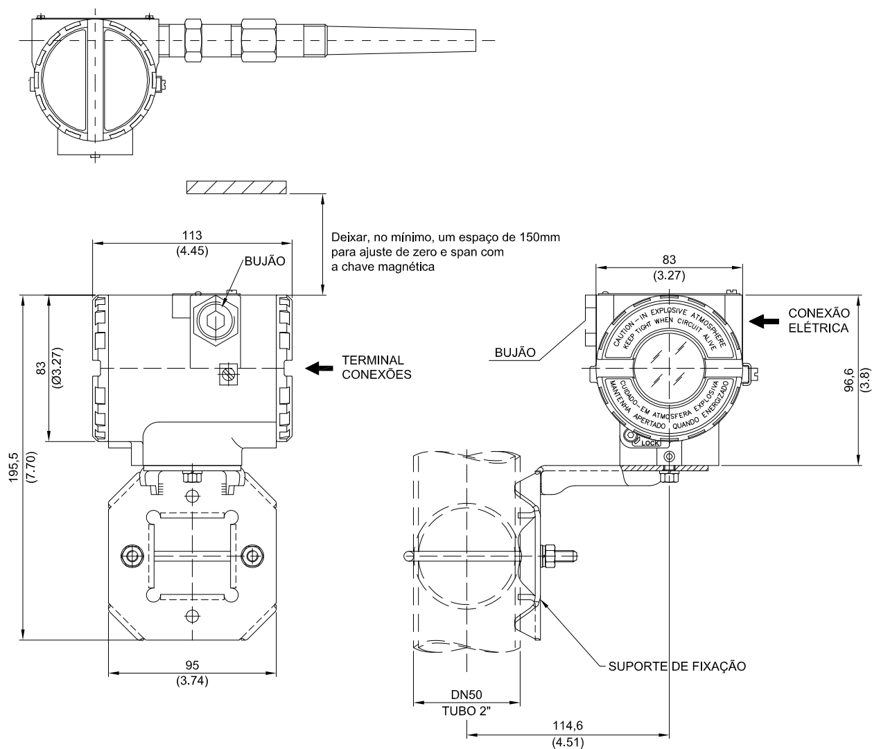
Figura 1.1 - Desenho Dimensional e Posições de Montagem
