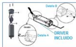
Figura 3 (Conexão eléctrica)
