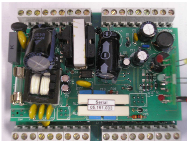
Figura A.1 – Vista superior do Multi-point (com uma chave de fenda, retire o parafuso)
