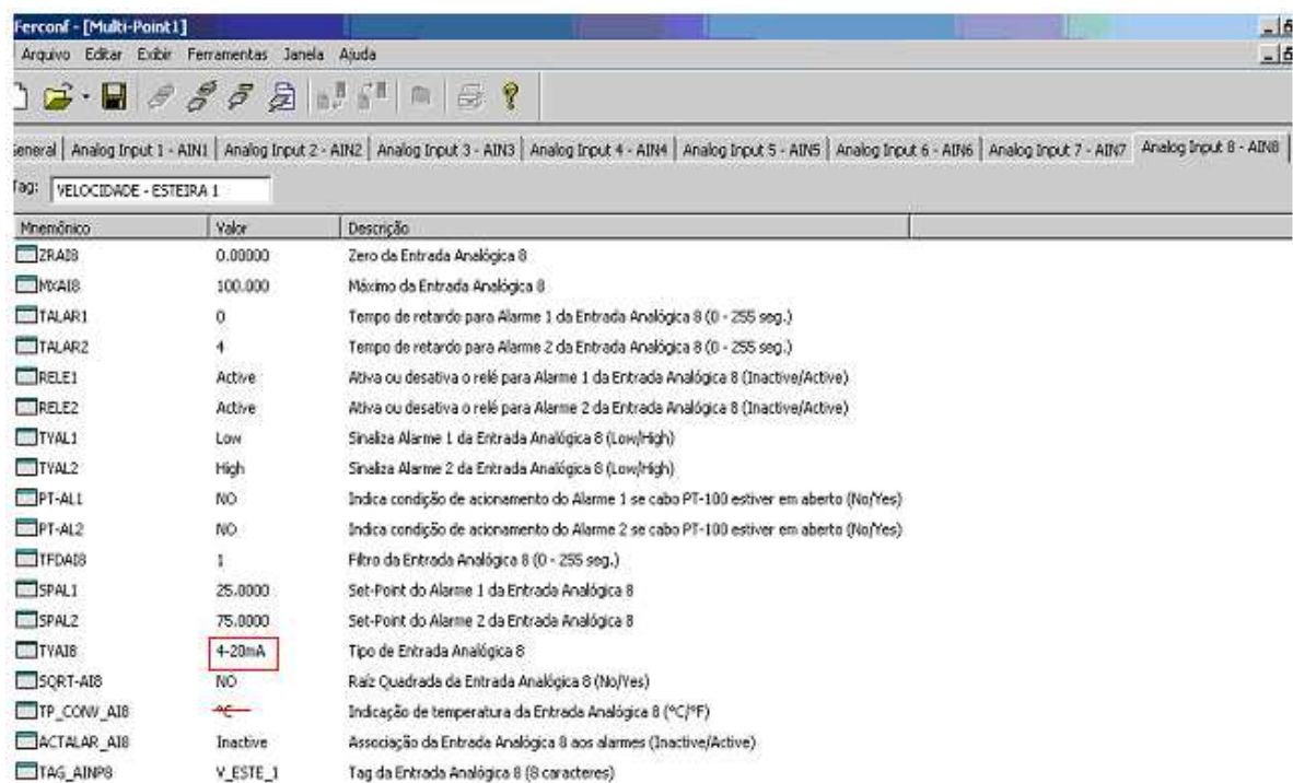
Figura II.9 – Tela de configuração de uma das entradas configurada para 4-20mA no Multi-Point
