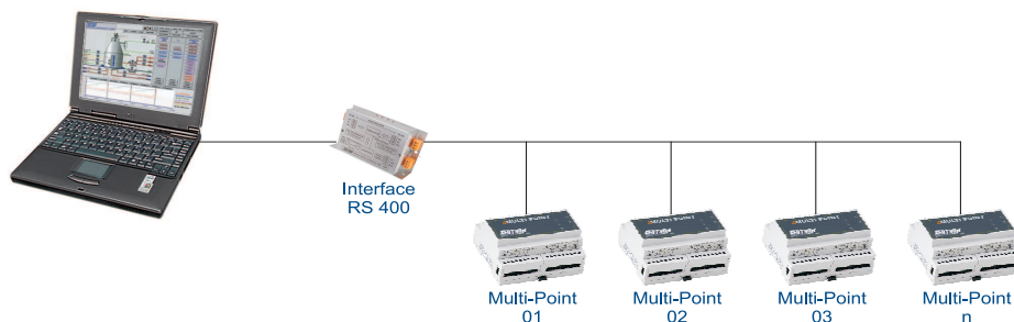
Figura II.2 - Configuração entre Micro, interface e Multi-point
