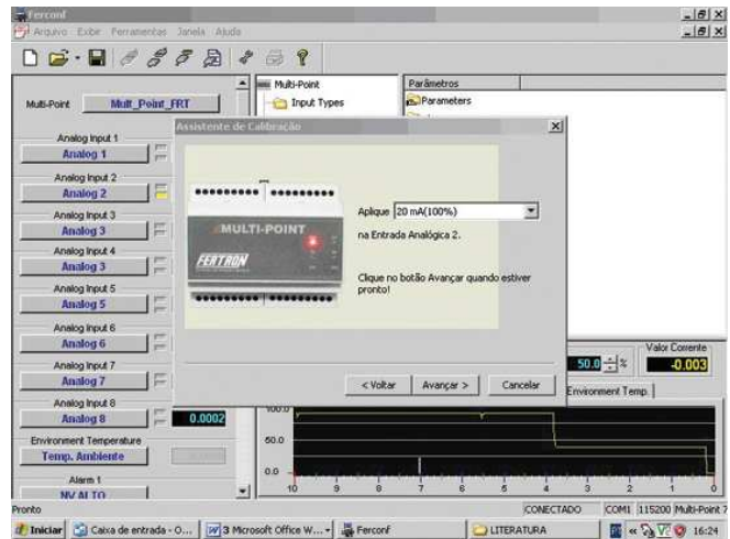
Figura B.3 – Assistente de Calibração (passo 3)
