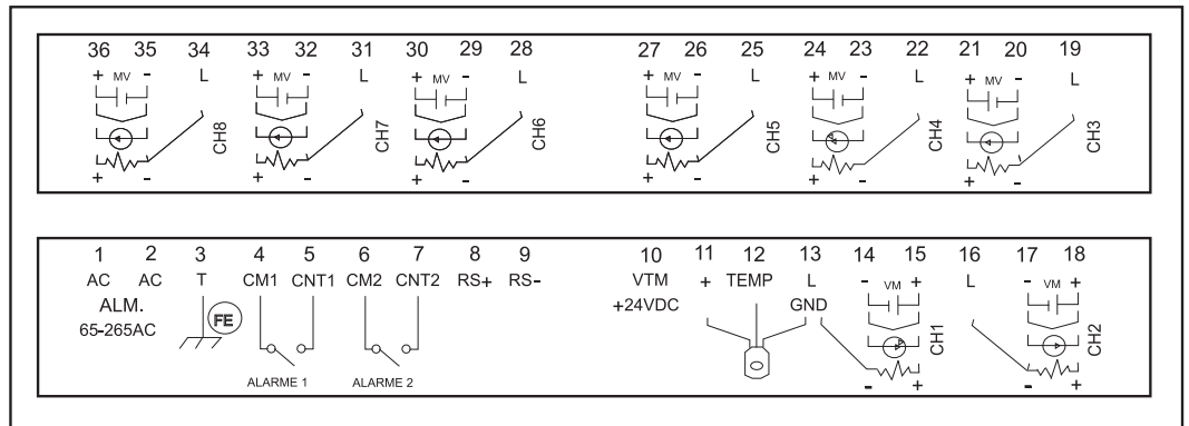
Figura II.6 - Ligações para os sensores de campo
