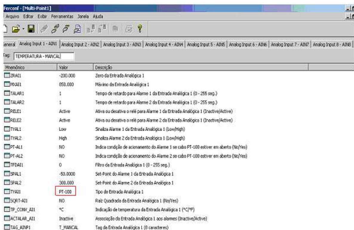
Figura II.8 – Tela de configuração de uma das entradas configurada para Pt-100 do Multi-Point
