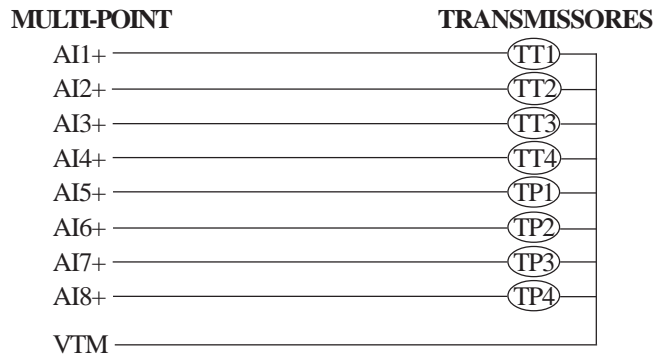
Figura II.7 - Alimentação de transmissores a dois fios
