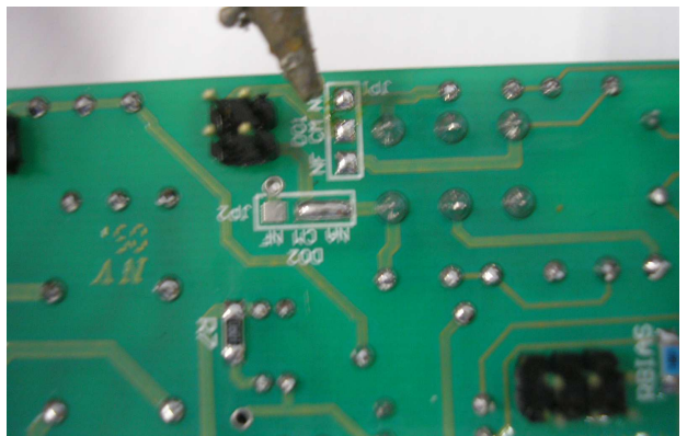
Figura A.4 – Com um ferro de solda e um sugador, retire o contato NA CM
