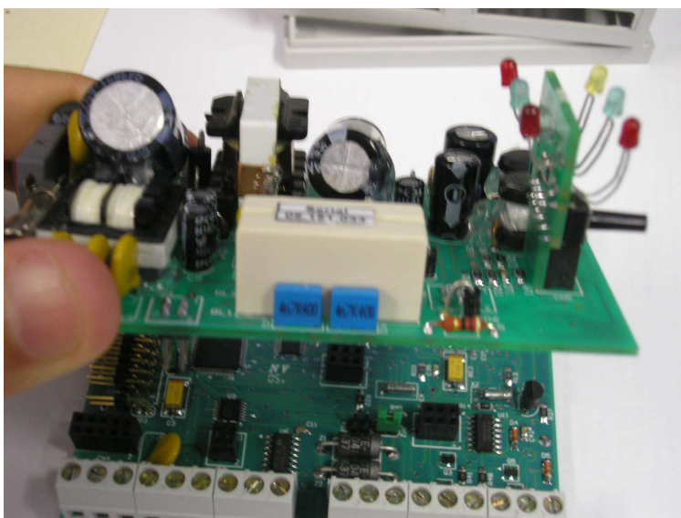
Figura A.2 – Retire a placa da fonte e relés
