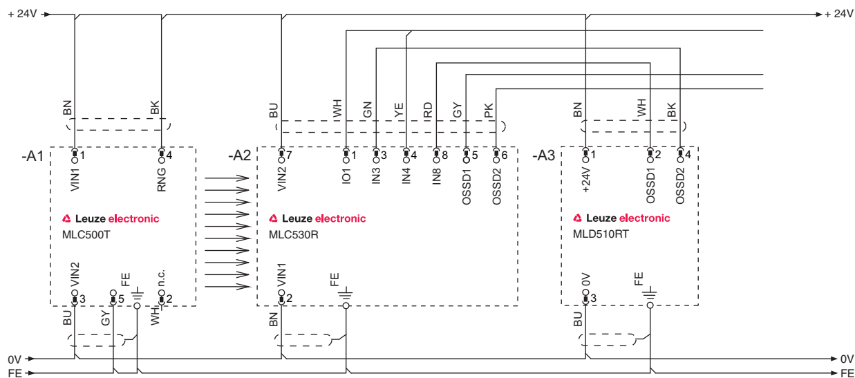
Ilustração 7.9: Modo de operação 2: exemplo de circuito para concatenação de saídas eletrônicas de chaveamento de segurança para o monitoramento combinado de acessos e áreas
