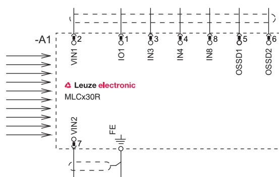
Ilustração 7.5:Diagrama de conexões do receptor
