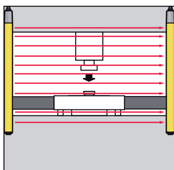
Ilustração 4.1: Blanking fixo: os bloqueios mecânicos previnem a intrusão na área de proteção pelos lados
