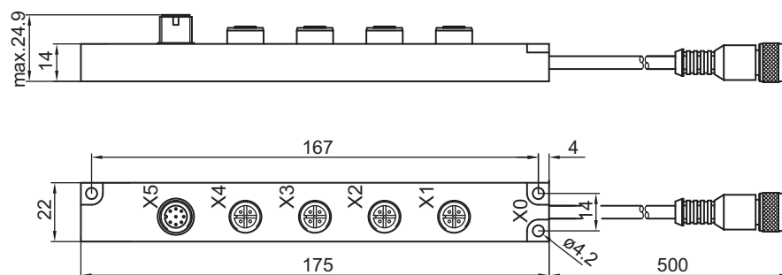
Ilustração 14.7: Módulo de conexão do sensor AC-SCM8
