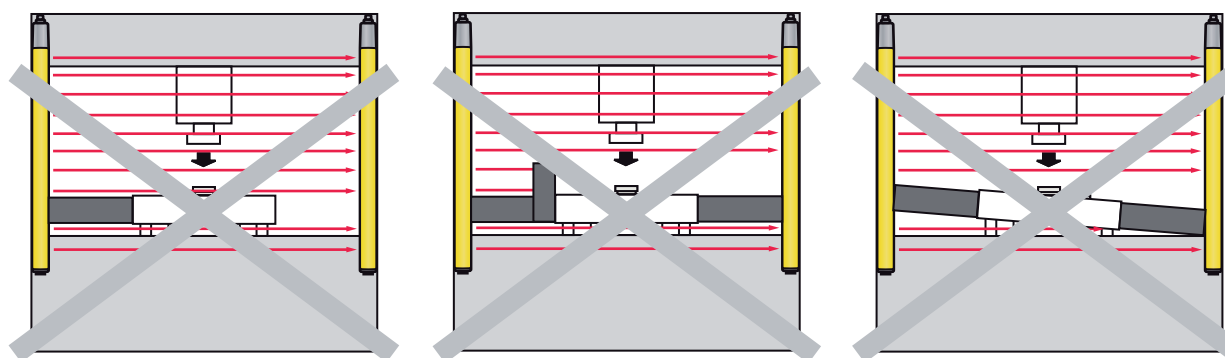
Ilustração 4.2: Blanking fixo: prevenção da “formação de sombras”
