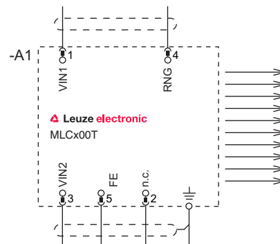
Ilustração 7.2: Diagrama de conexões do emissor
