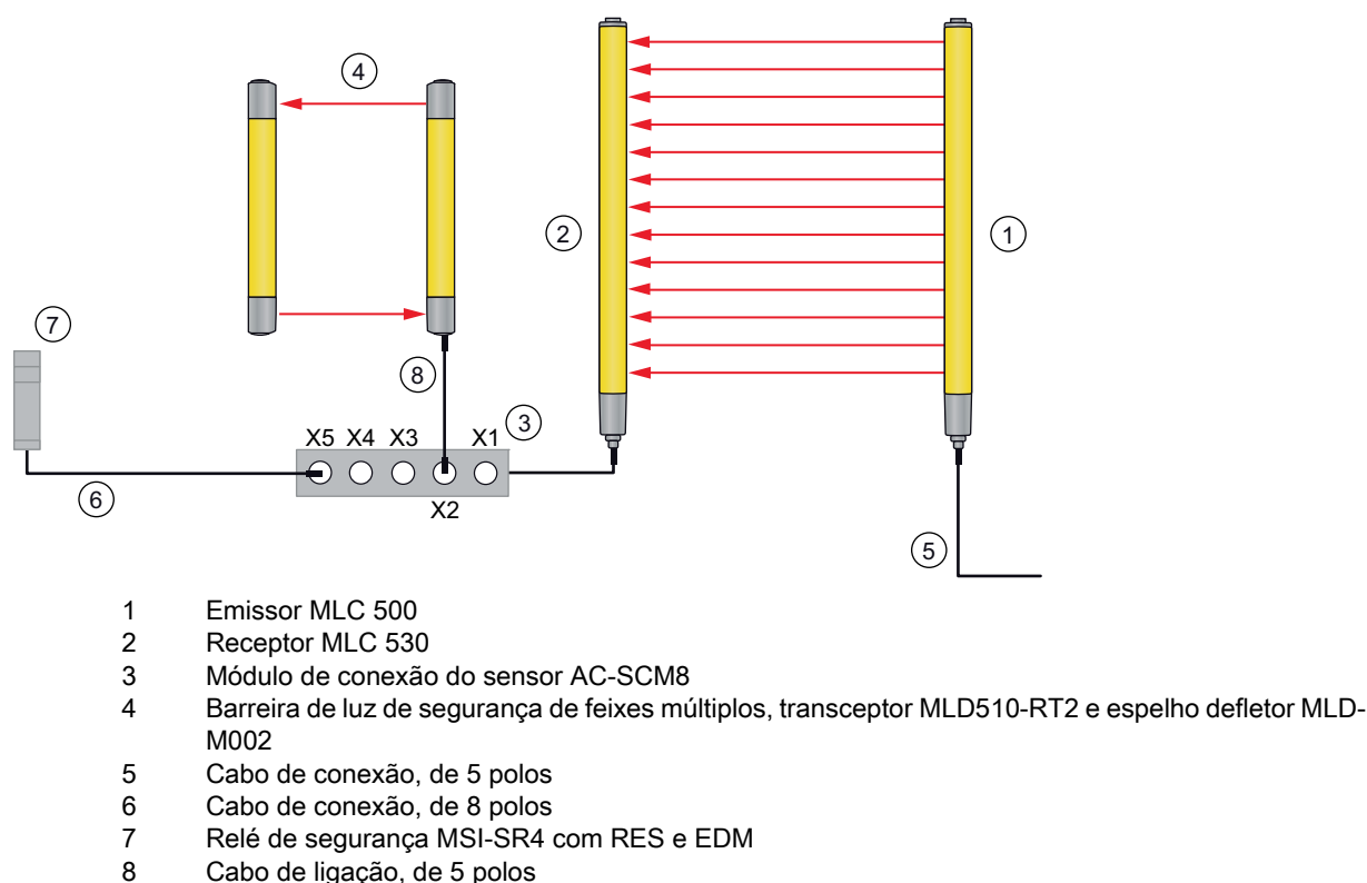
Ilustração 7.10: Modo de operação 2: exemplo de ligação com MLC 530 e MLD 510 para combinação de proteção de pontos de perigo e proteção de acesso
