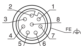
Ilustração 7.4:Ocupação dos conectores do receptor
