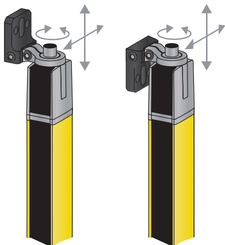
Ilustração 6.12: Montagem através de suporte giratório BT-R
