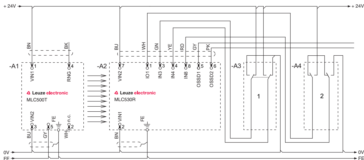
Ilustração 7.6: Modo de operação 1: exemplo de circuito para concatenação com interruptor de posição para monitoramento da presença de peças de máquinas escondidas
