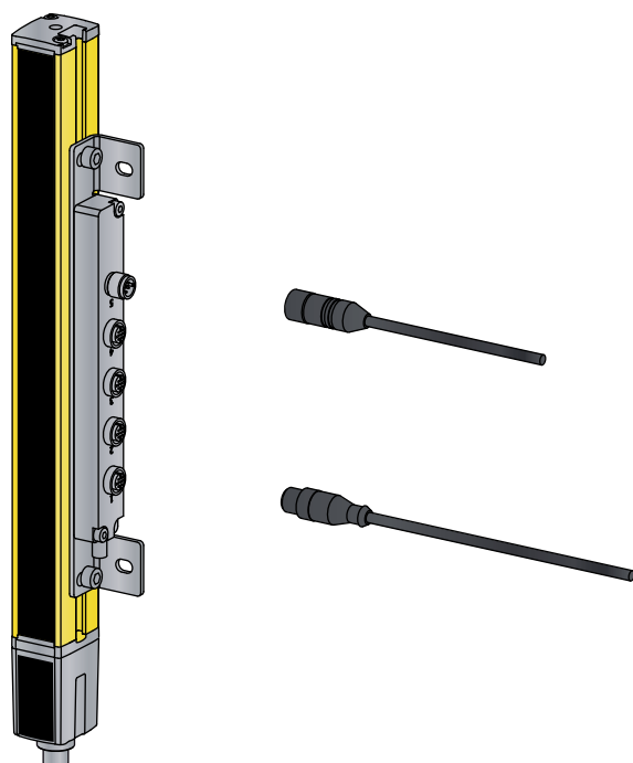
Ilustração 6.15: Possibilidades de montagem do AC-SCM8-BT
