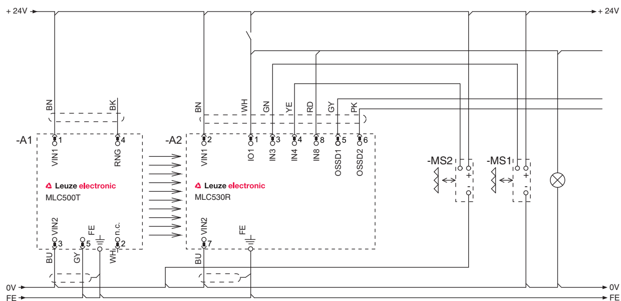
Ilustração 7.13: Modo de operação 4: exemplo de circuito para o muting temporal de 2 sensores
