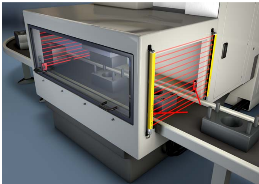
Ilustração 5.4: Proteção de acesso a pontos de perigo com muting
