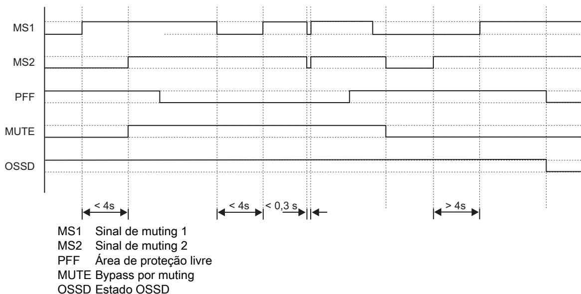
Ilustração 4.6: Muting temporal - transcurso de tempo
