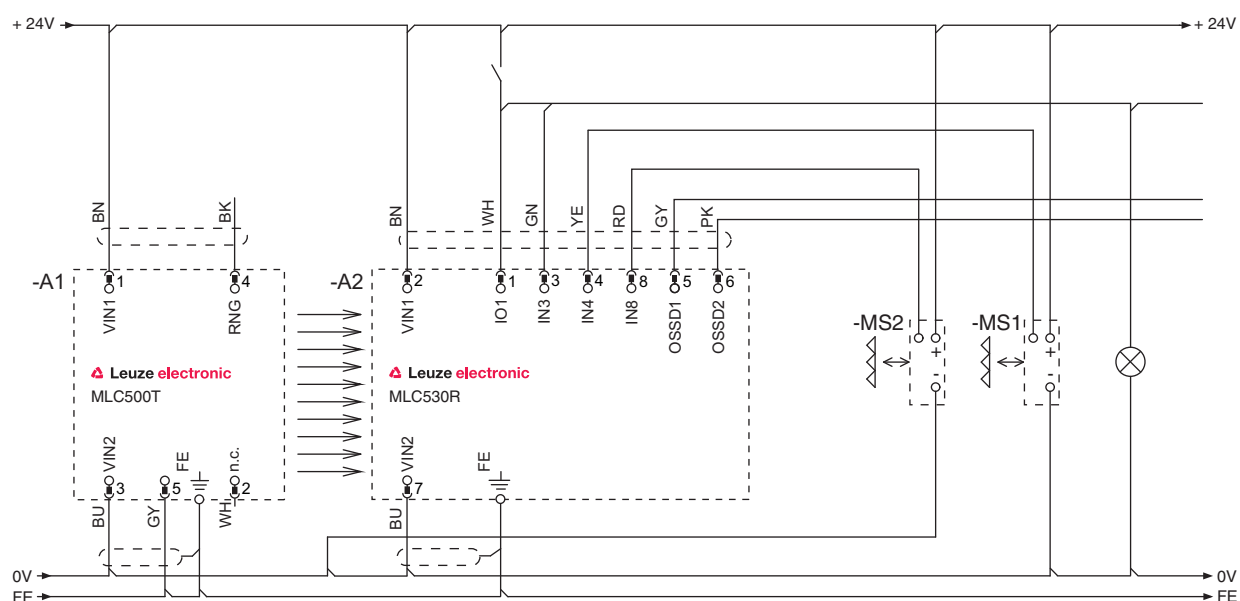
Ilustração 7.15: Modo de operação 6: exemplo de circuito com muting temporal de 2 sensores (parcial)
