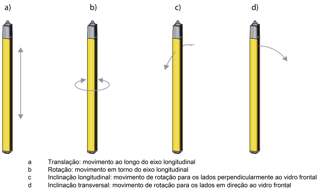
Ilustração 6.10: Sentidos de movimento para o alinhamento do sensor de segurança
