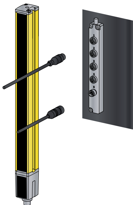
Ilustração 6.14: Possibilidades de montagem do AC-SCM8
