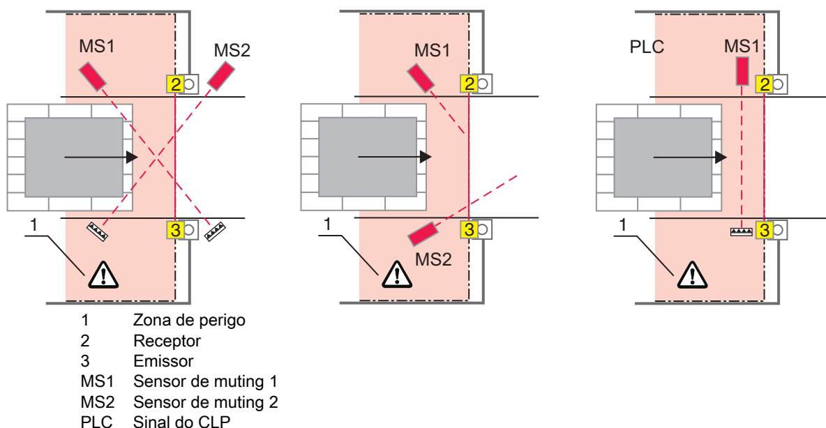
Ilustração 6.9: Disposição do sensor de muting no caso de muting temporal de 2 sensores em uma aplicação de saída
