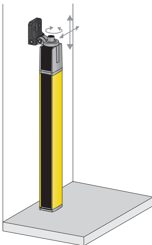
Ilustração 6.13: Fixação diretamente à bancada da máquina
