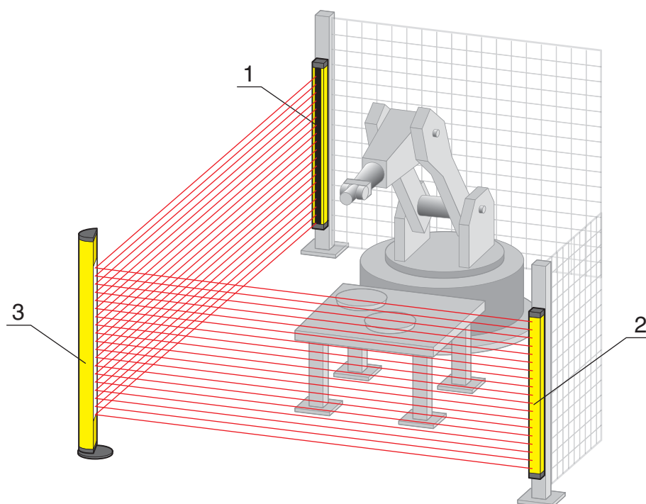
Ilustração 6.16: Disposição com espelho defletor para uma proteção de um ponto de perigo em dois lados
