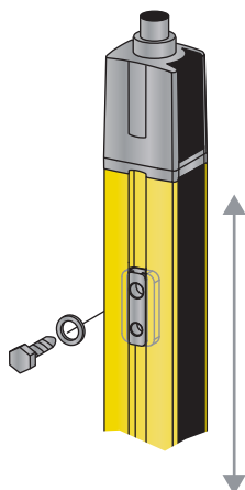
Ilustração 6.11: Montagem através de porcas para ranhuras em T BT-NC60
