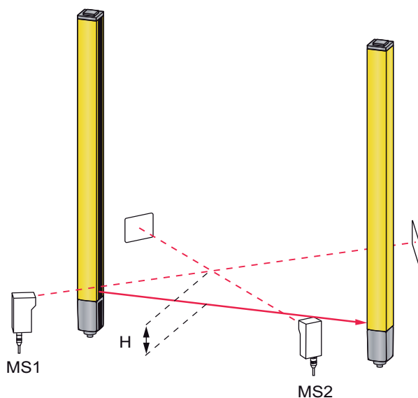
Ilustração 6.8: Disposição dos sensores de muting na altura
