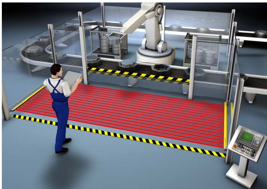
Ilustração 5.5: Proteção de acesso a zonas de perigo em um robô
