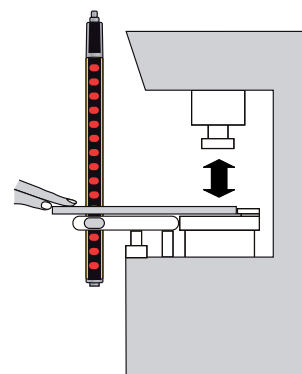
Ilustração 4.4: Resolução reduzida; diversos objetos suficientemente pequenos podem ser movidos, ao mesmo tempo, dentro da área de proteção ou ser removidos
