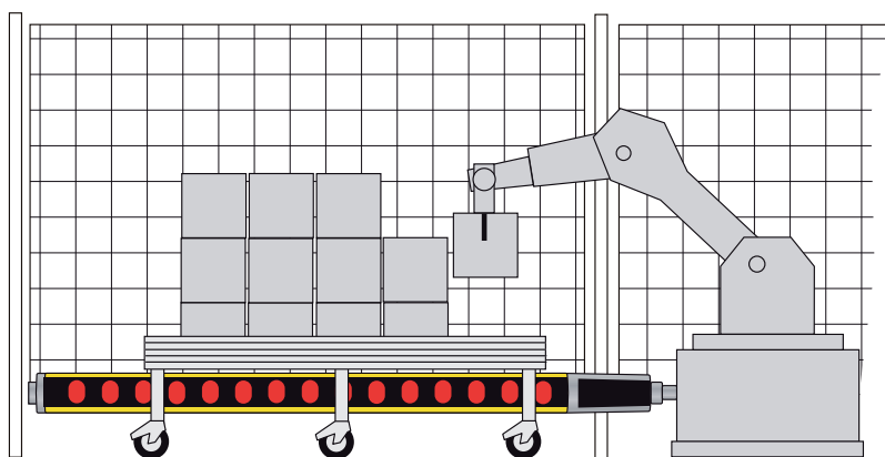
Ilustração 4.4: Resolução reduzida; diversos objetos suficientemente pequenos podem ser movidos, ao mesmo tempo, dentro da área de proteção ou ser removidos
