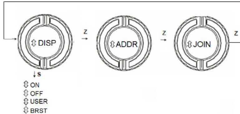
Figura 2.5 – Opções para ajuste local
