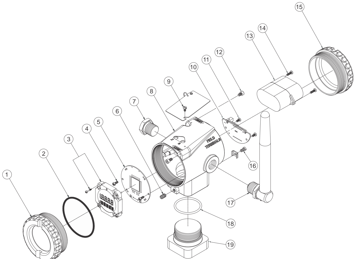
Figura 3.3 – Desenho Explodido
