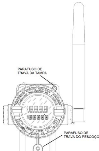
Figura 1.6 – Parafusos de Ajuste da Carcaça e Trava da Tampa
