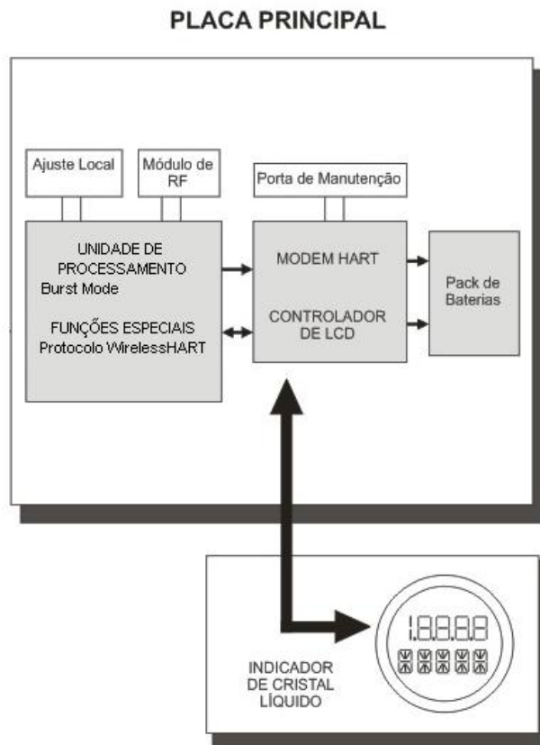
Figura 2.1 - Diagrama de Blocos do RP400 WirelessHART ®
