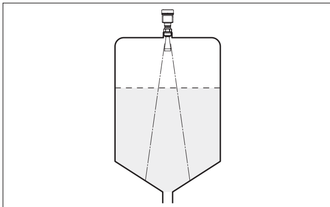
Fig. 6: Montagem do sensor de radar em reservatórios com fundo cônico
