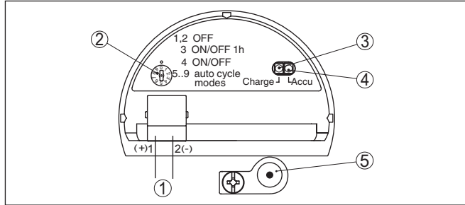
Fig. 24: Compartimento de alimentação
