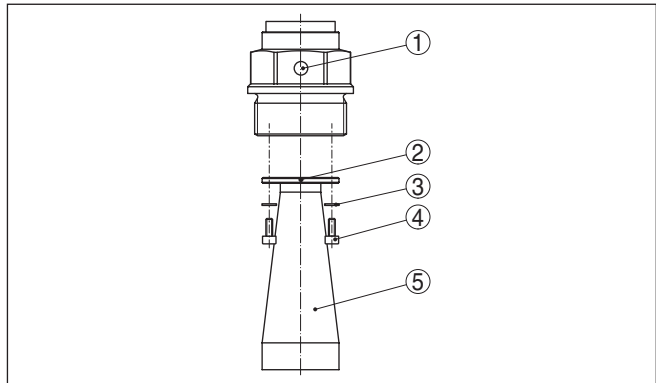
Fig. 2: Desmontagem da antena tipo corneta
