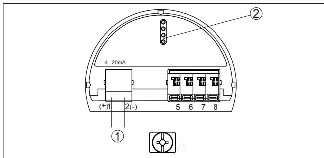
Fig. 23: Compartimento do sistema eletrônico da caixa de duas câmaras
