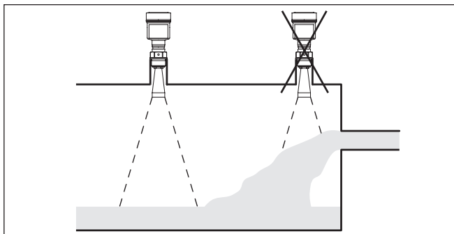
Fig. 7: Montagem do sensor de radar no fluxo de entrada do produto
