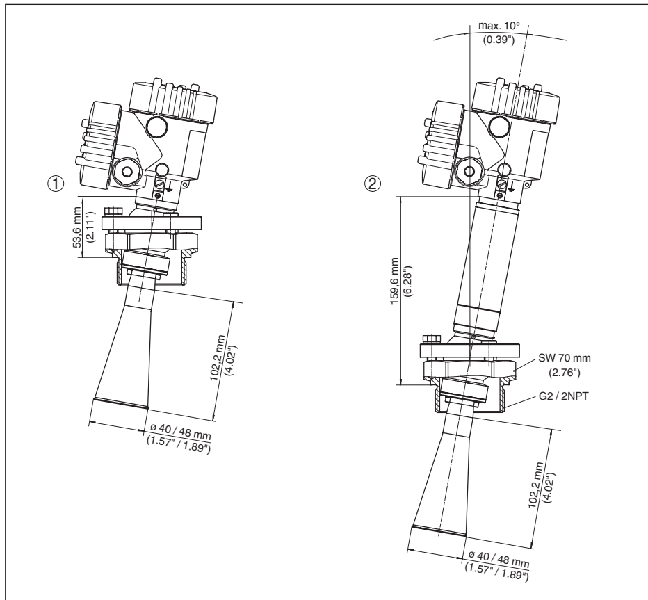
Fig. 55: VEGAPULS 62, antena tipo corneta e suporte giratório, conexão roscada
