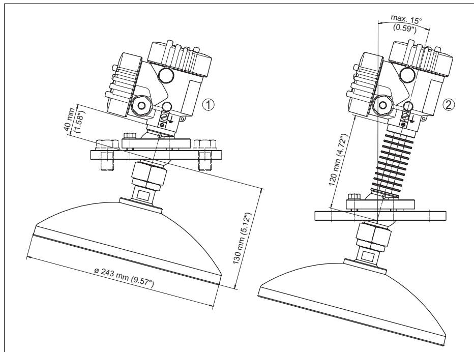
Fig. 56: VEGAPULS 62, antena parabólica e suporte giratório
