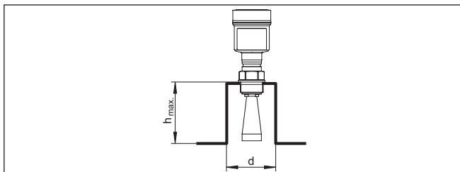
Fig. 12: Medidas diferentes da luva
