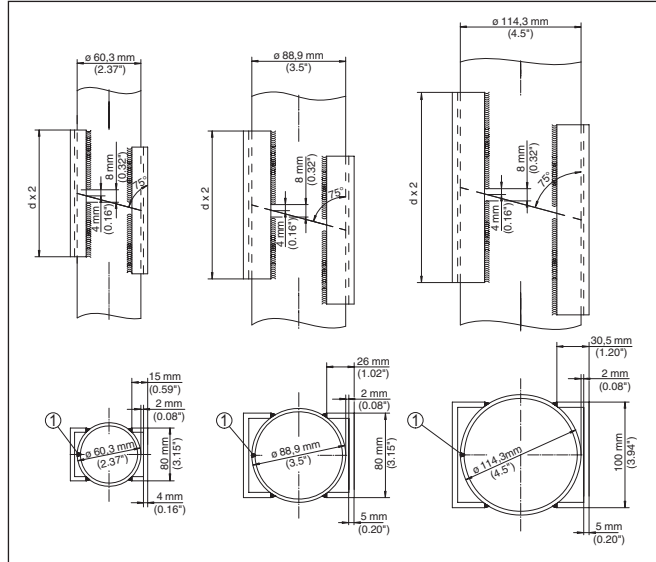
Fig. 18: União soldada no prolongamento do tubo tranquilizador para diferentes exemplos de diâmetro
