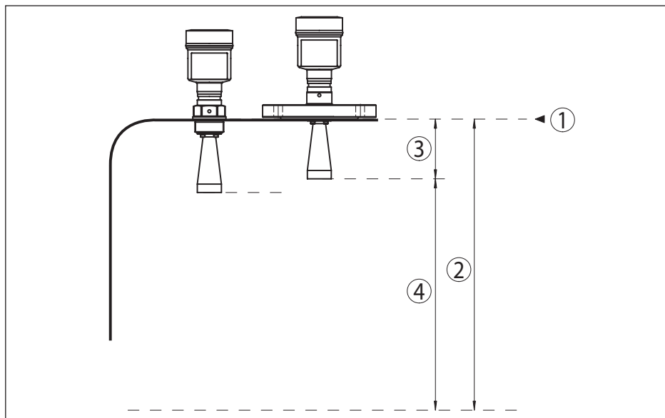
Fig. 47: Dados referentes à grandeza de entrada
