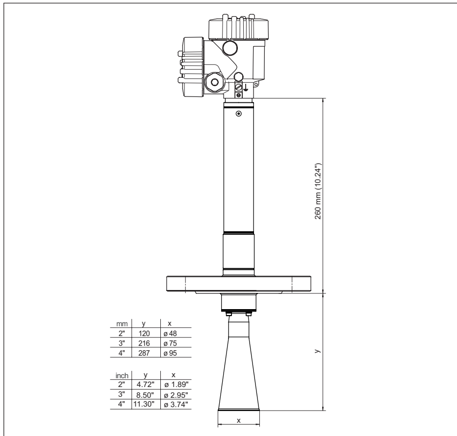
Fig. 53: VEGAPULS 62, Antena tipo corneta em modelo com flange com adaptador de temperatura até 450 °C
