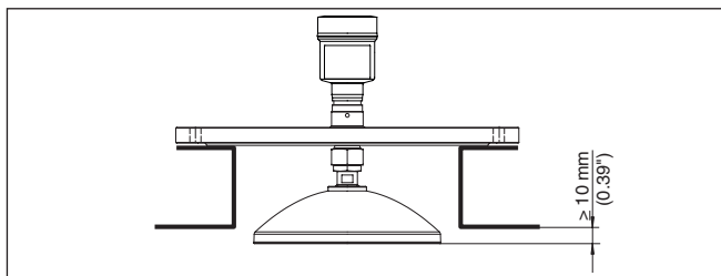
Fig. 9: Montagem recomendada em luva de tubo no caso de antena parabólica
