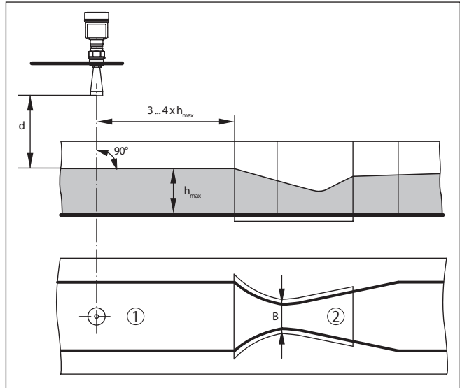
Fig. 21: Medição de débito com calha tipo Venturi Khafagi; d = distância mínima do sensor; h_{max} = enchimento máx. da calha; B = maior estreitamento da calha
