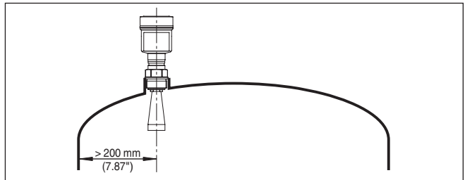
Fig. 5: Montagem do sensor de radar em teto de reservatório redondo
