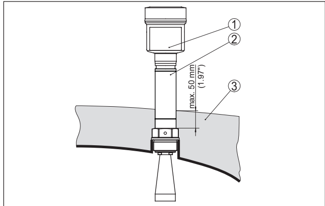
Fig. 16: Montagem do aparelho em reservatórios isolados.
