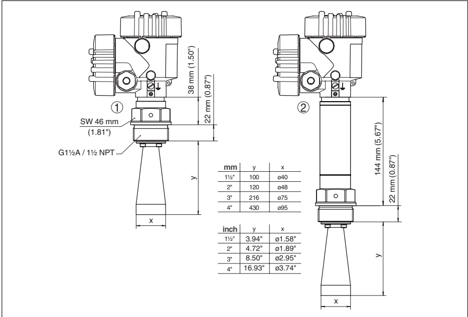
Fig. 50: VEGAPULS 62, antena tipo corneta em modelo com rosca
