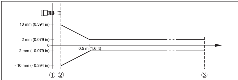
Fig. 48: Diferença de medição sob condições de referência
