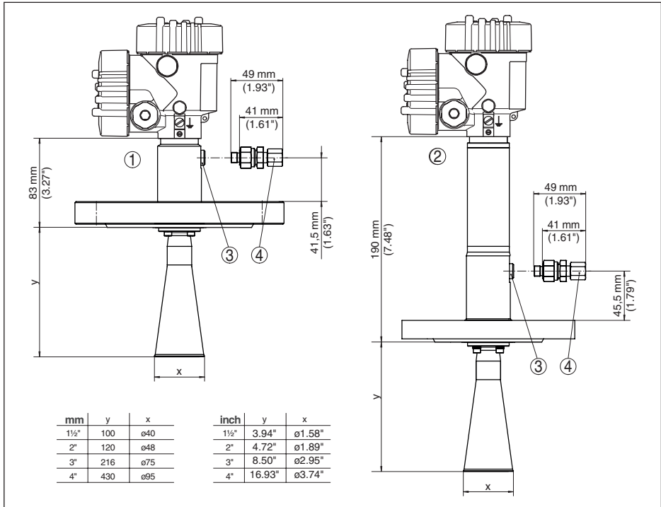
Fig. 52: VEGAPULS 62, Antena tipo corneta em modelo com flange e conexão de ar de limpeza
