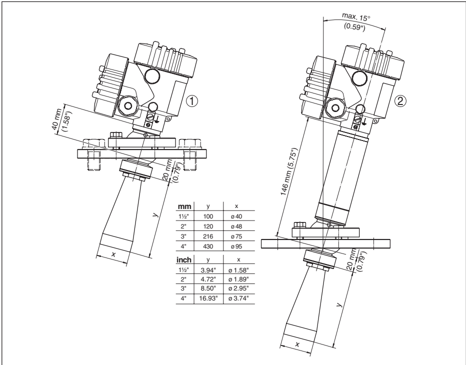
Fig. 54: VEGAPULS 62, antena tipo corneta e superte rotativo
