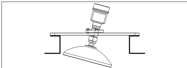
Fig. 11: Distância entre antena e luva no caso de antena parabólica
