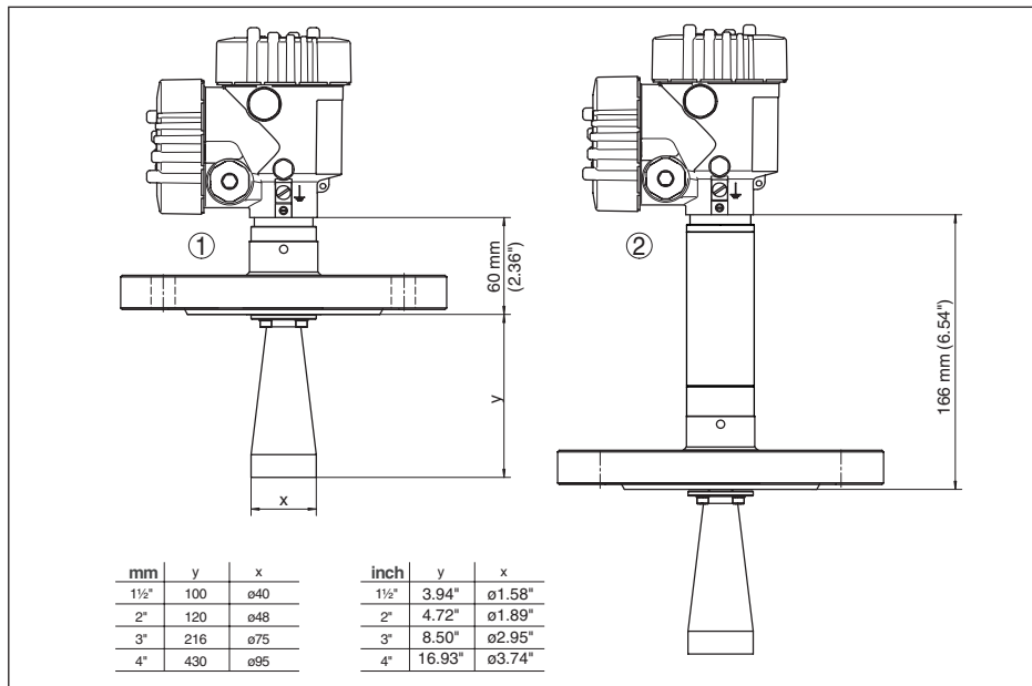
Fig. 51: VEGAPULS 62, antena em forma de chifre em modelo com flange
