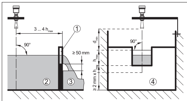
Fig. 20: Medição de débito com calha retangular: d_{min} = distância mínima do sensor (vide capítulo "Dados técnicos"); h_{max} = enchimento máx. da calha retangular
