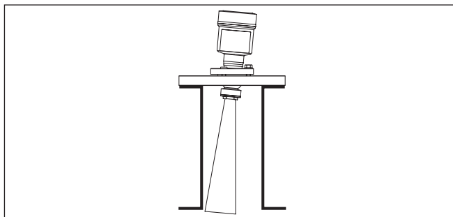
Fig. 10: Distância entre antena e luva no caso de antena tipo corneta
