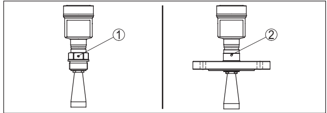
Fig. 4: Posição da polarização
