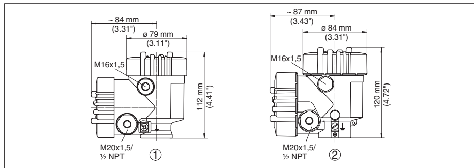
Fig. 49: Dimensões da caixa - com o módulo de visualização e configuração, a altura da caixa é aumentada em 9 mm/0.35 in
