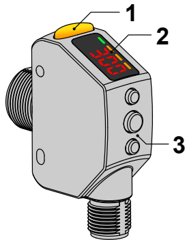
Figura 1: Recursos do Sensor
