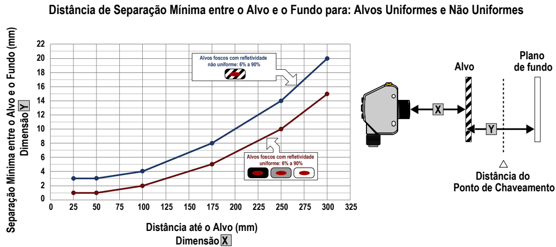
Figura 10: Distância de Separação Mínima de Objetos (90% a 6% de refletância)
