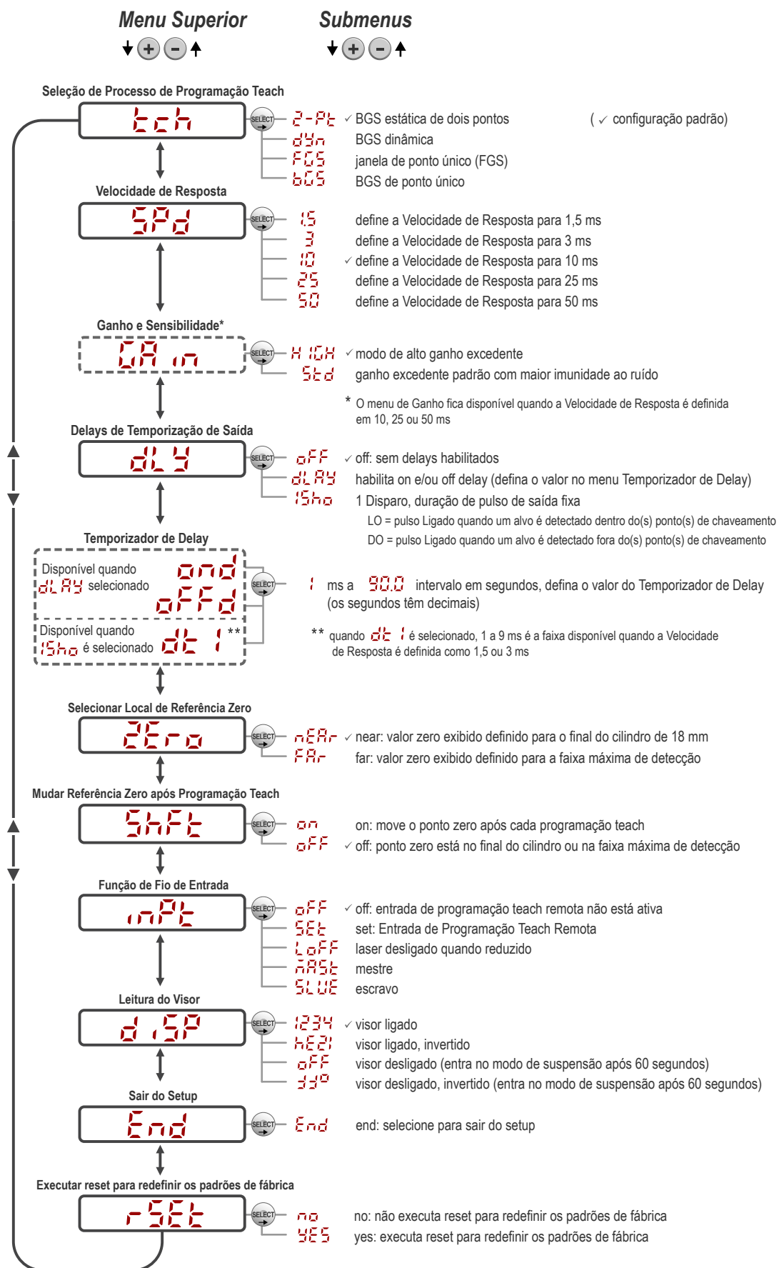
Figura 9: Mapa de Menus do Sensor
