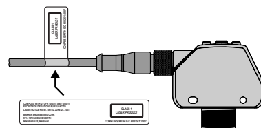
Figura 3: Instalação do Rótulo de Segurança
