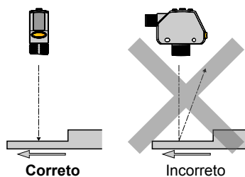
Figura 7: Orientação para uma diferença de altura
